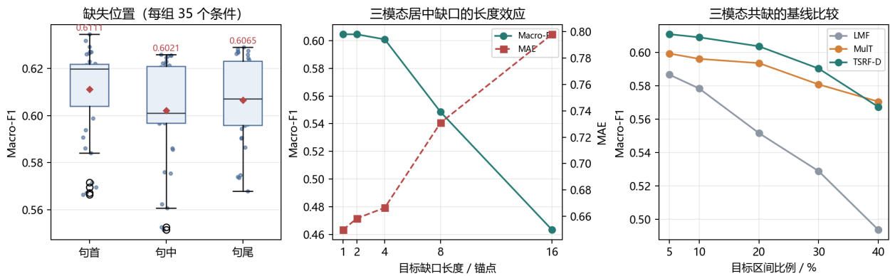
图 13 缺失位置、缺口长度与基线比较
