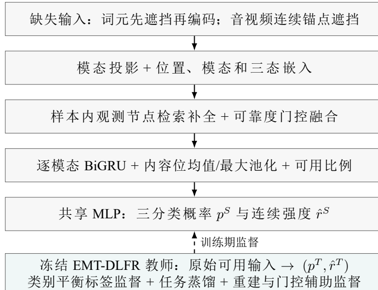
图 10 TSRF-D 网络结构与教师-学生监督关系
