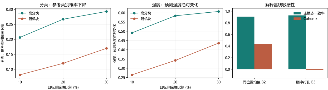
图 21 冻结测试子集上的分类与强度删除验证及解释基线敏感性
