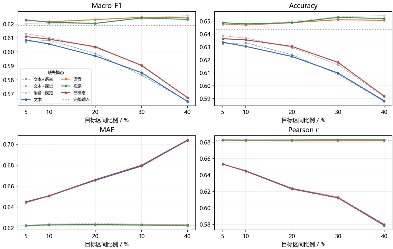
图 12 不同缺失模态与目标区间比例下四项指标的退化曲线
