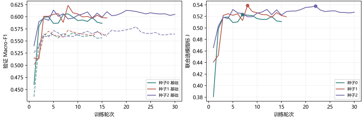
图 11 三个学生种子的训练过程
