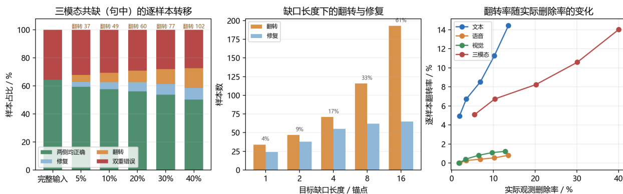
图 14 受控缺口下的逐样本错误转移
