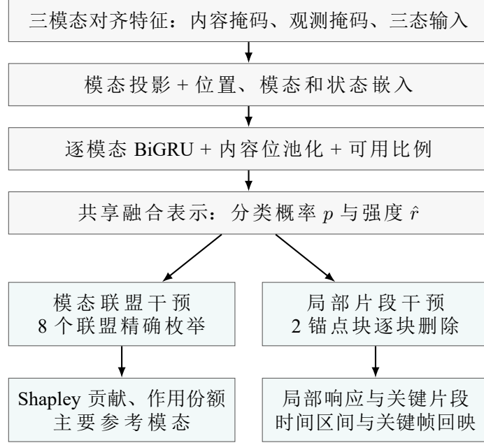
图 18 问题三 ICF-Shapley 预测器与解释层结构
