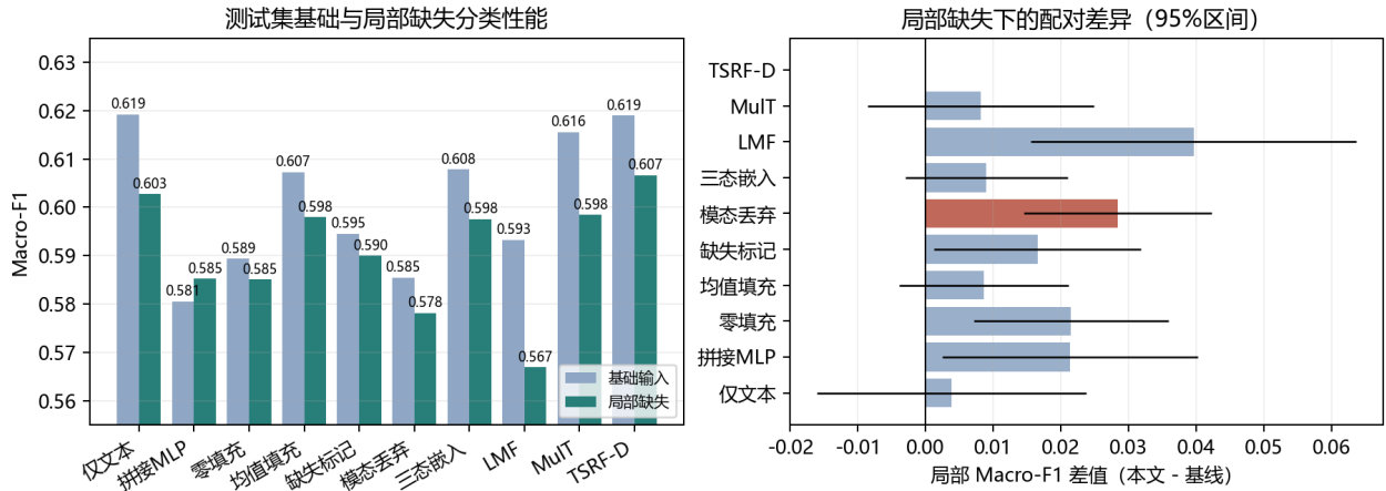
图 16 十类模型在测试集上的比较
