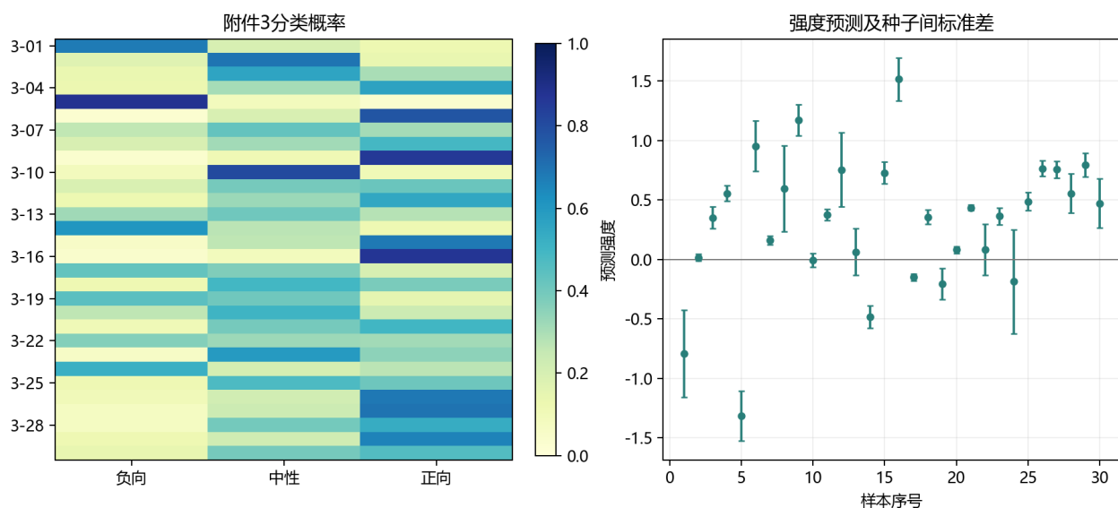
图 17 附件 3 全量样本的分类概率与强度预测
