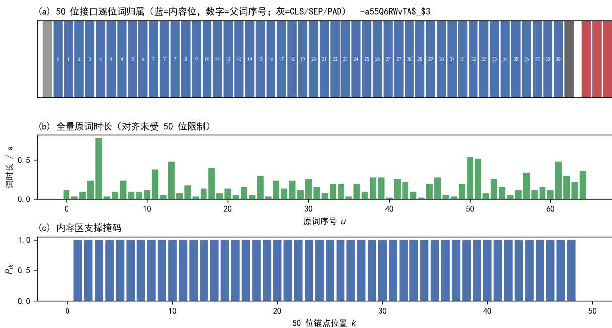
图 8 样本-a55Q6RWvTA$_$3 的文本接口截断
