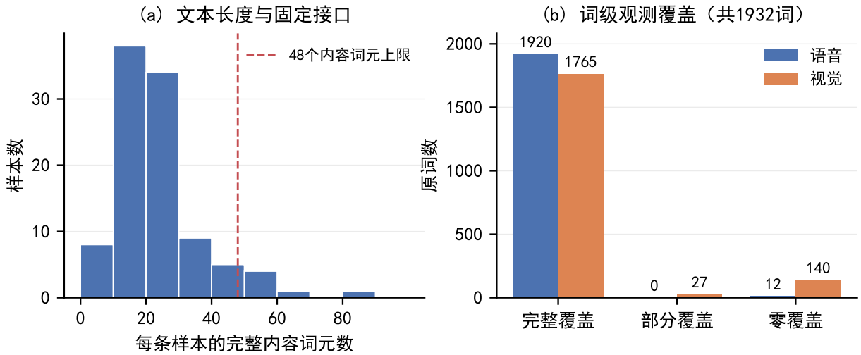
图 5 由样本清单和词级明细重算的接口覆盖情况
