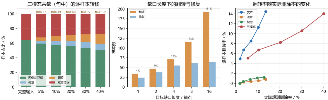
图 13 受控缺口下的逐样本错误转移
