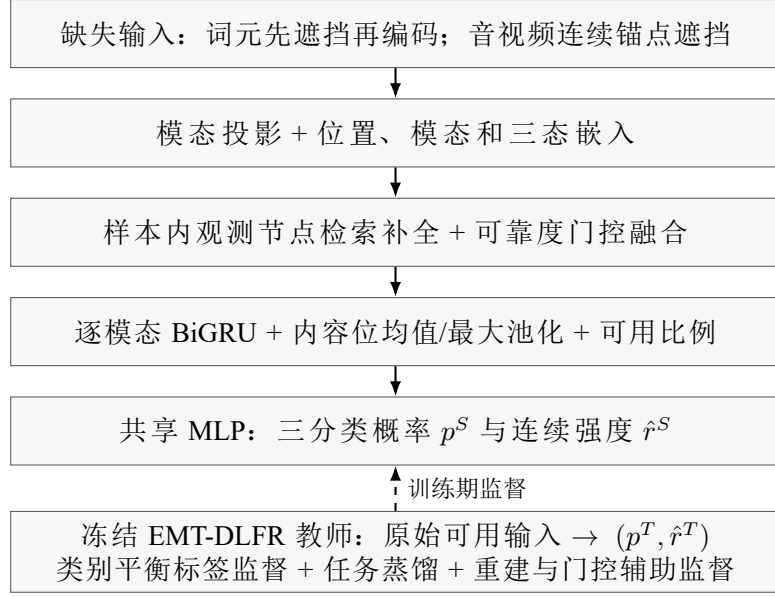
图9 TSRF-D 网络结构与教师-学生监督关系
