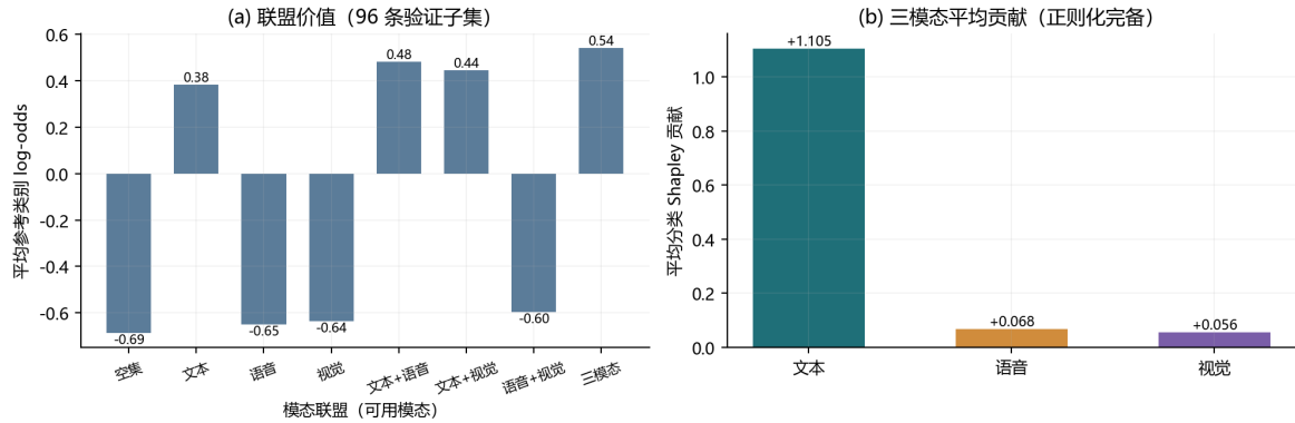
图 20 模态联盟的平均分类价值与三模态平均 Shapley 贡献。
