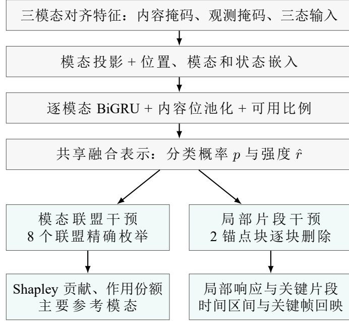
图 18 问题三 ICF-Shapley 预测器与解释层结构。两类干预均调用同一冻结预测器，分别产生模态级和片段级解释。
