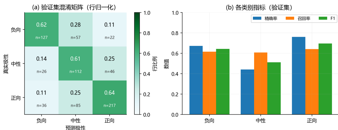
图 19 验证集混淆矩阵与分类指标。
