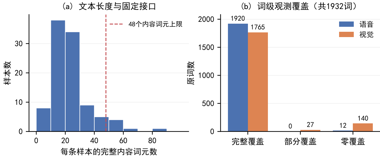
图 5 由样本清单和词级明细重算的接口覆盖情况。左图为 100 条样本的完整词元数，虚线表示 48 个内容词元上限；6 条样本触发截断，共 70 个词元未进入接口。右图以全部 1932 个原词为分母，区分完整、部分与零覆盖；完整覆盖按 d \geq 1 - 10^{-6} 判定。
