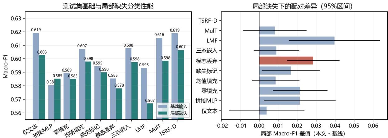
图 16 十类模型在测试集上的比较。(a) 基础输入与 105 种连续局部缺失条件下的 Macro-F1；(b) 局部条件下本文模型相对各基线的配对差异及 95% 区间，红色表示经 Holm 校正后达到 5% 显著性水平。
