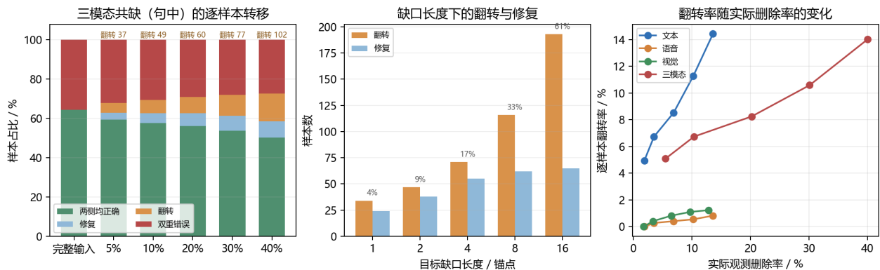
图 14 受控缺口下的逐样本错误转移。(a) 三模态居中缺口的四类样本占比与翻转样本数；(b) 缺口长度下的翻转与修复样本数，顶部标注实际观测删除率；(c) 各模态组合的翻转率随实际删除率的变化。
