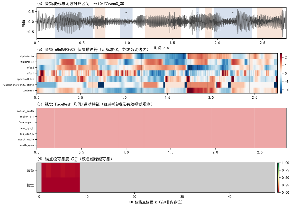
图 7 局部视觉观测缺失样本。上三幅以秒为横轴，下方质量条带以 50 位接口索引为横轴，二者通过父词映射和词区间关联。红带表示视觉无效帧（未检出或相邻帧运动不可测），灰色接口位置为非内容位。
