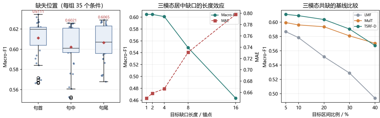
图 13 缺失位置、缺口长度与基线比较。(a) 各位置 35 个连续缺失条件的 Macro-F1 分布与组均值；(b) 三模态居中缺口的长度曲线；(c) 三模态共缺下三个模型的 Macro-F1 比较。
