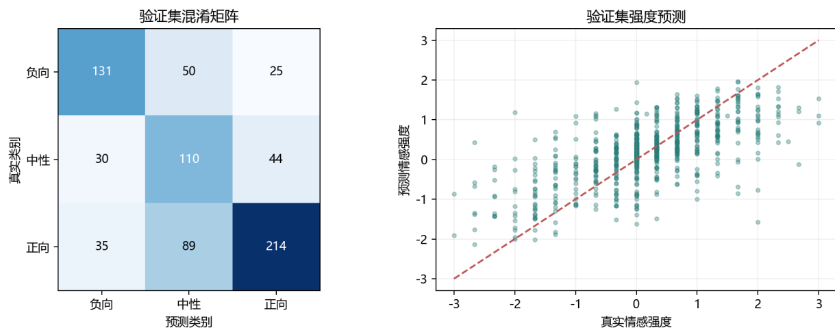
图 15 验证集类别混淆与强度回归结果。
