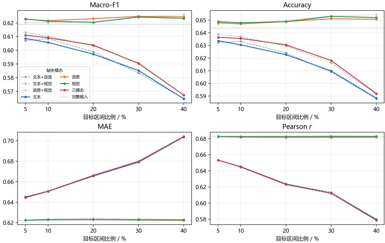
图 12 不同缺失模态与目标区间比例下四项指标的退化曲线。单模态与三模态共缺为实线，双模态组合为浅色虚线，点线为完整输入水平。
