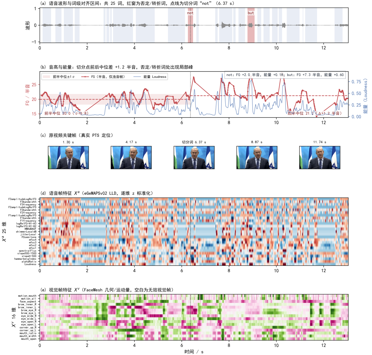
图 6 典型样本的文本、语音与视频对应。五层共用同一秒轴：(a) 波形与全部词区间，红窗为否定/转折词；(b) F_0 （半音，仅浊音帧）与能量包络，虚线为前、后半段中位，点线为切分词时刻；(c) 按真实 PTS 定位的关键帧；(d) 25 维语音帧特征；(e) 16 维视觉帧特征。热图的逐维标准化仅用于可视化。
