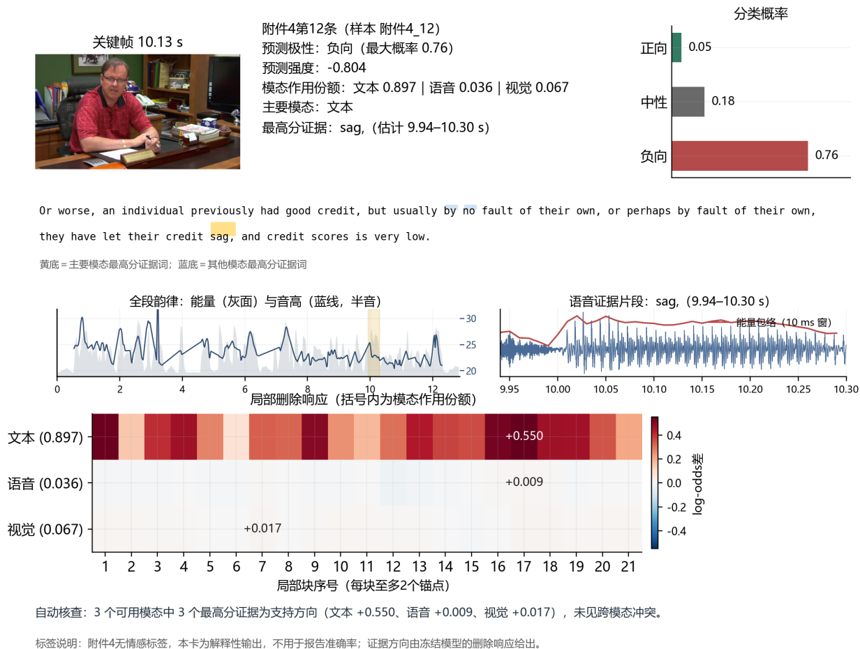
图 23 附件 4 第 12 条 (转折样本) 解释卡。自上而下依次为原始关键帧、预测与模态份额、分类概率、原文证据高亮、全段韵律轨迹、语音证据波形与逐块删除响应; 份额由绝对 Shapley 贡献归一化得到, 响应为删除前后参考类别的 log-odds 差, 正值表示支持。
