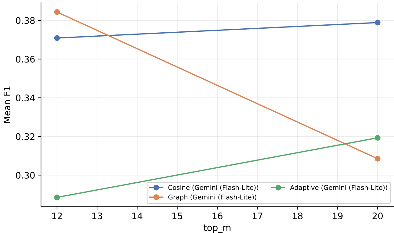
F1 vs. top_m - 2WIKI
