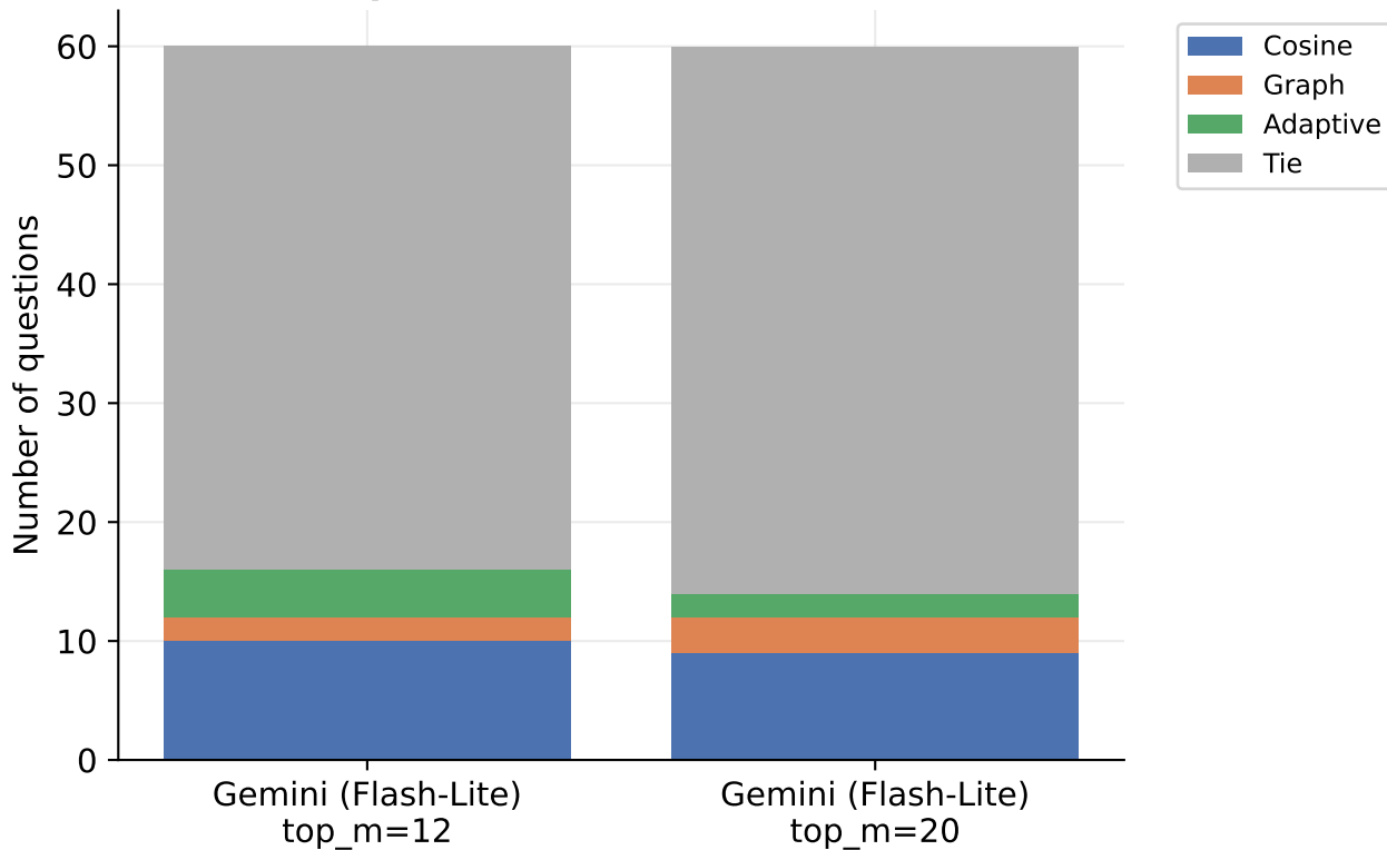
Per-question F1 winner - MUSIQUE
