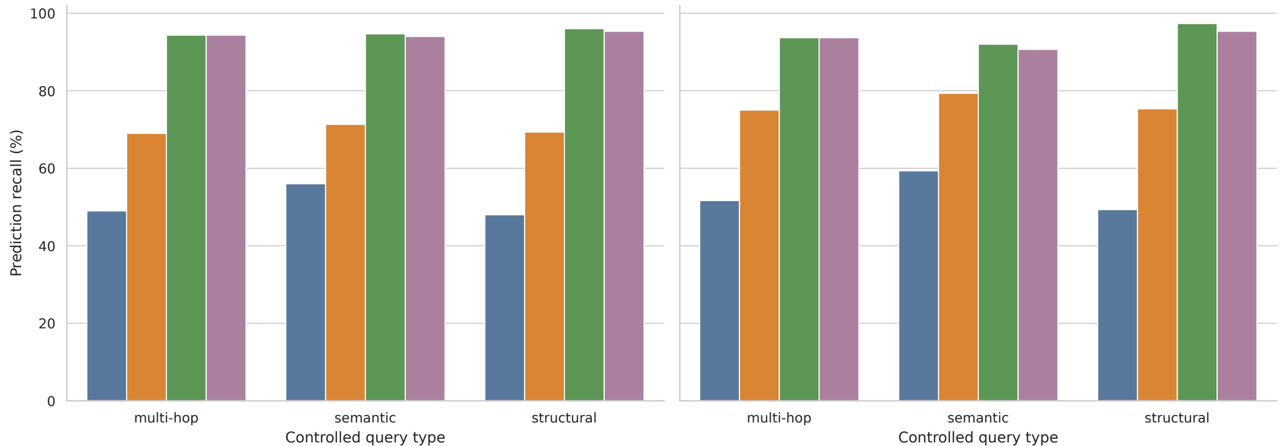
Qwen-2.5-1.5B
