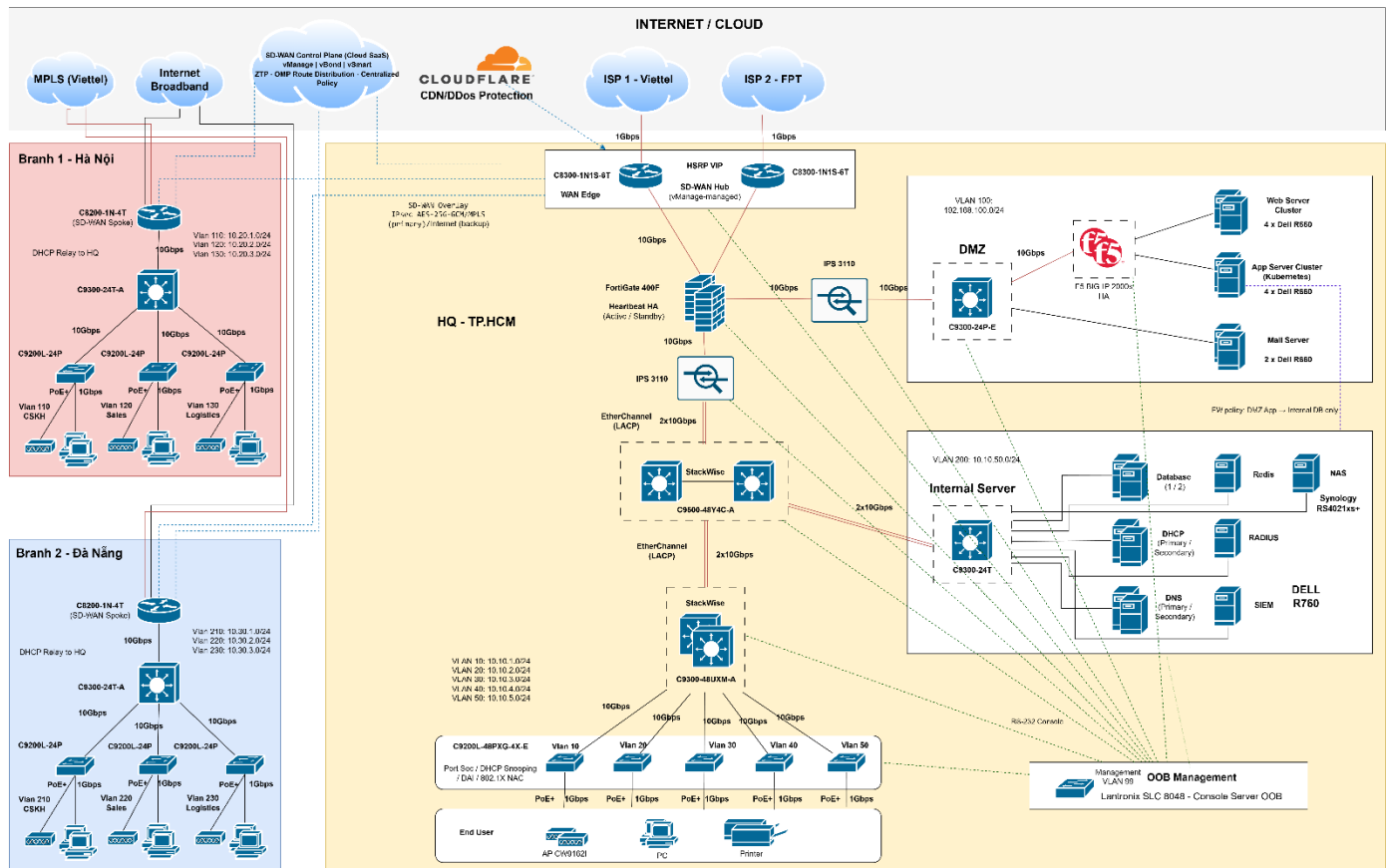
Hình 1: Sơ đồ luận lý toàn hệ thống Otech
