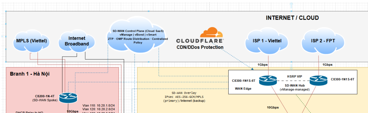
Hình 3: Kiến trúc SD-WAN HQ Hub – Branch Spoke
