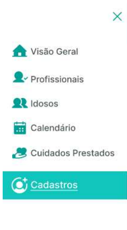
Figura 7 – Componente Menu(Maximizado)
