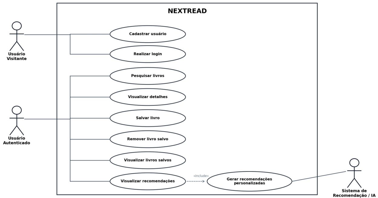
Figura 1 - Diagrama de casos de uso do NextRead.
