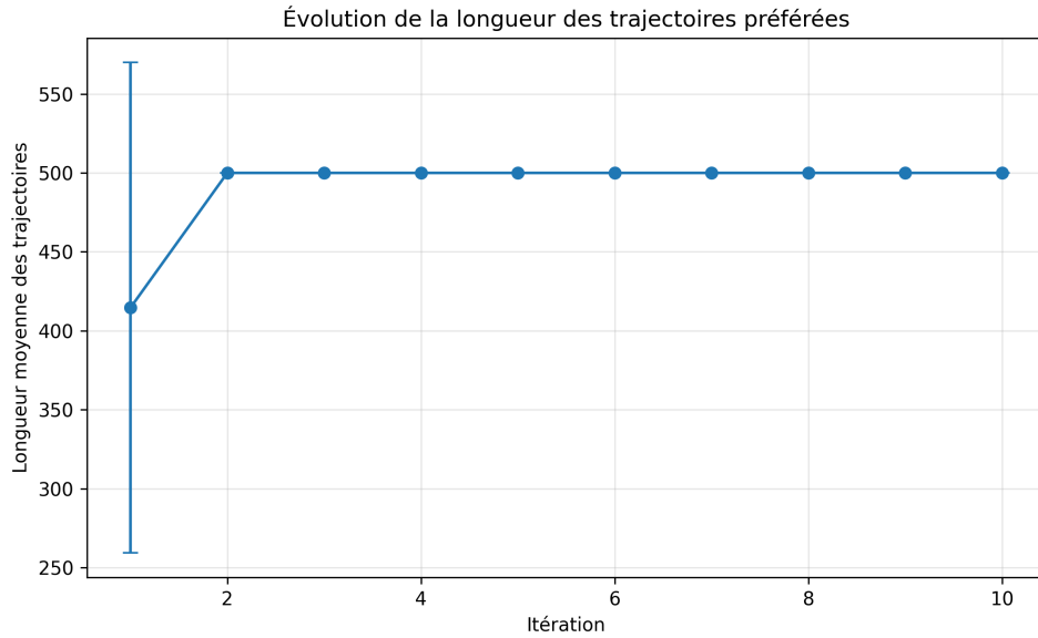
FIGURE 3 – Evolution de la longueur des trajectoires préférées
