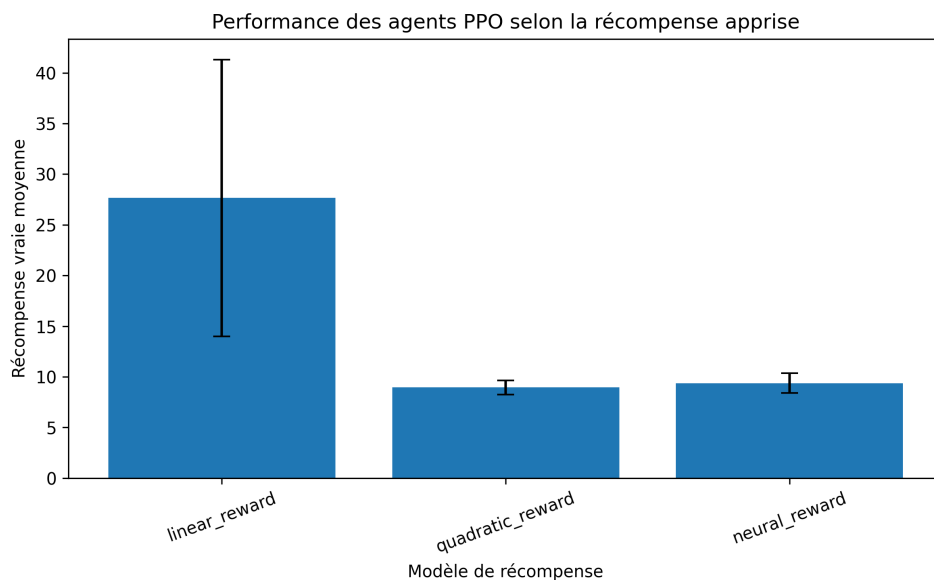
FIGURE 2 – Performance des agents PPO entraînés avec les récompenses apprises par discrimination état par état.
