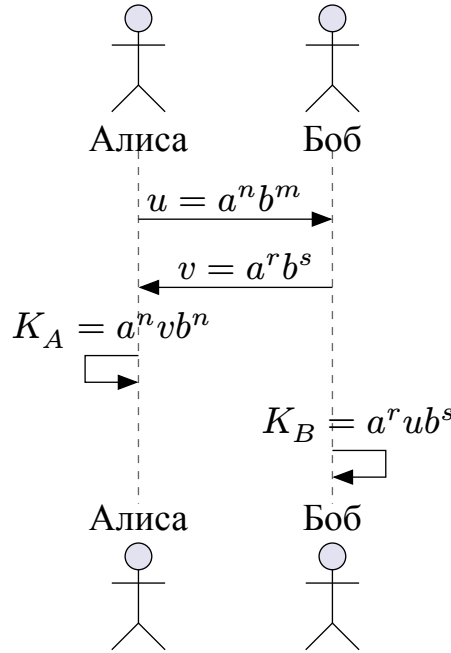
Рис. 1. Протокол Стикеля
