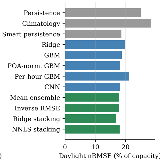
Rolling-origin
