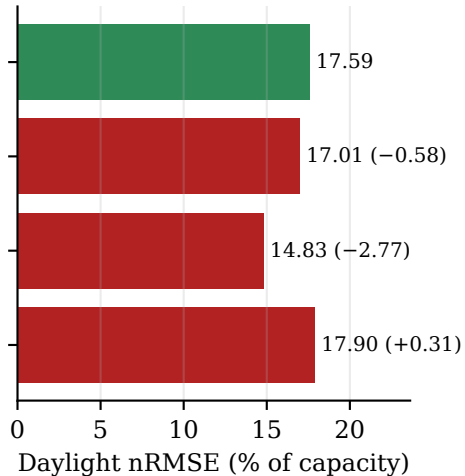
Rolling-origin
