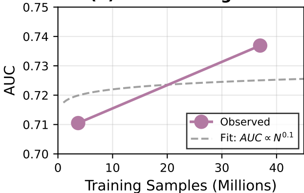
(d) Data Scaling Law
