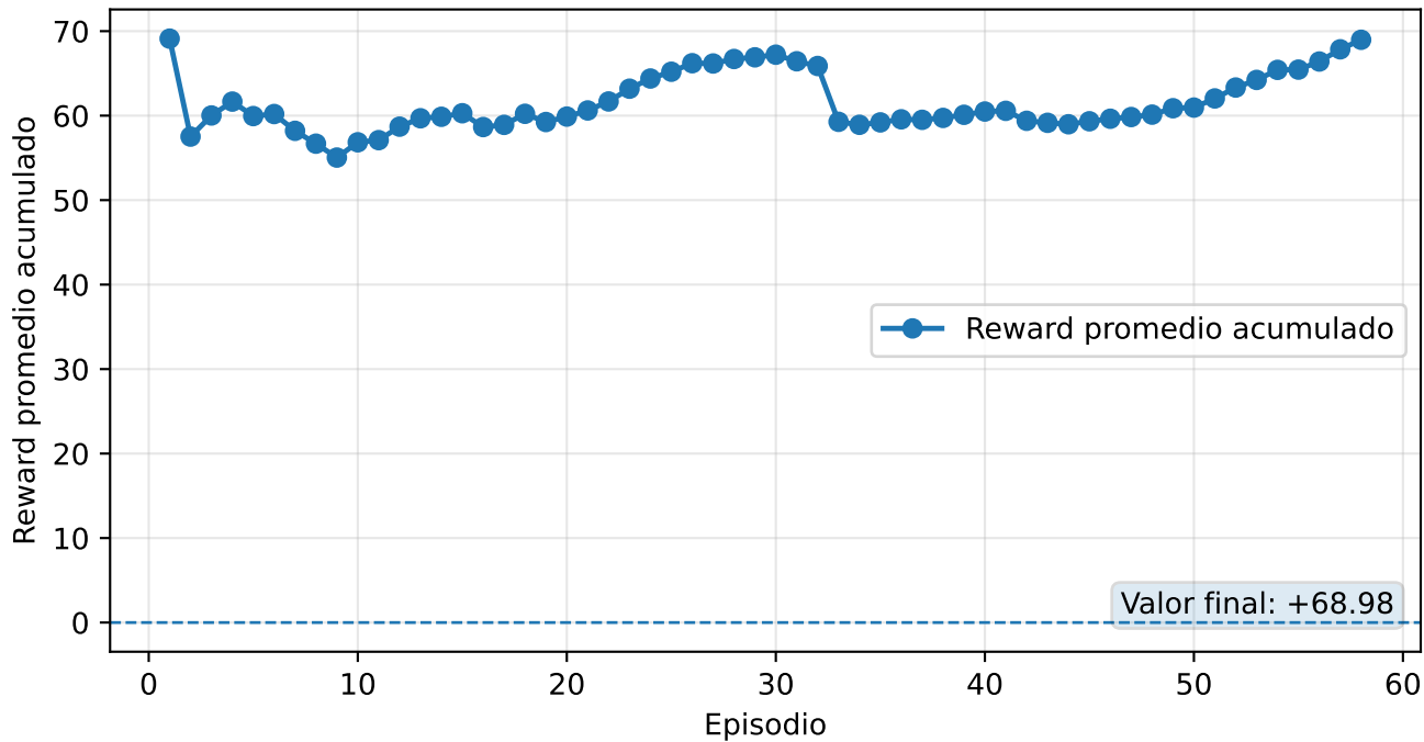
Reward promedio acumulado durante el entrenamiento
