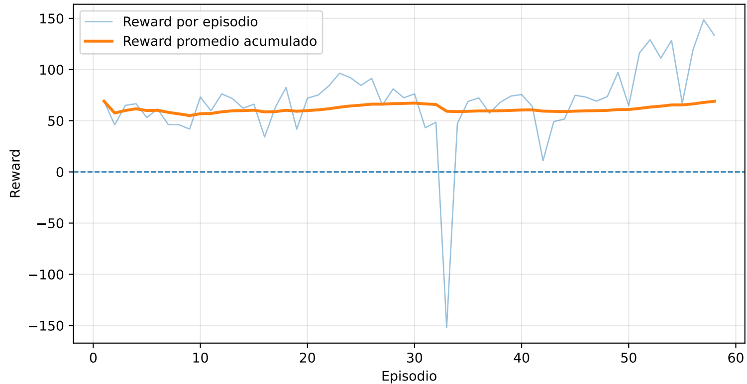
Reward de entrenamiento PPO
