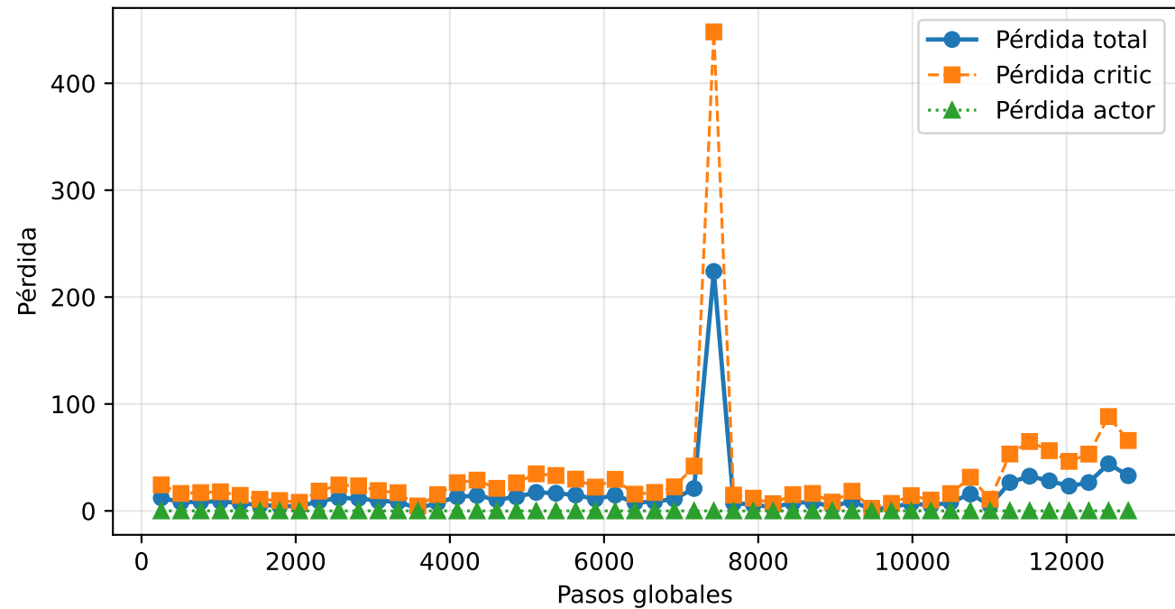
Componentes de pérdida PPO
