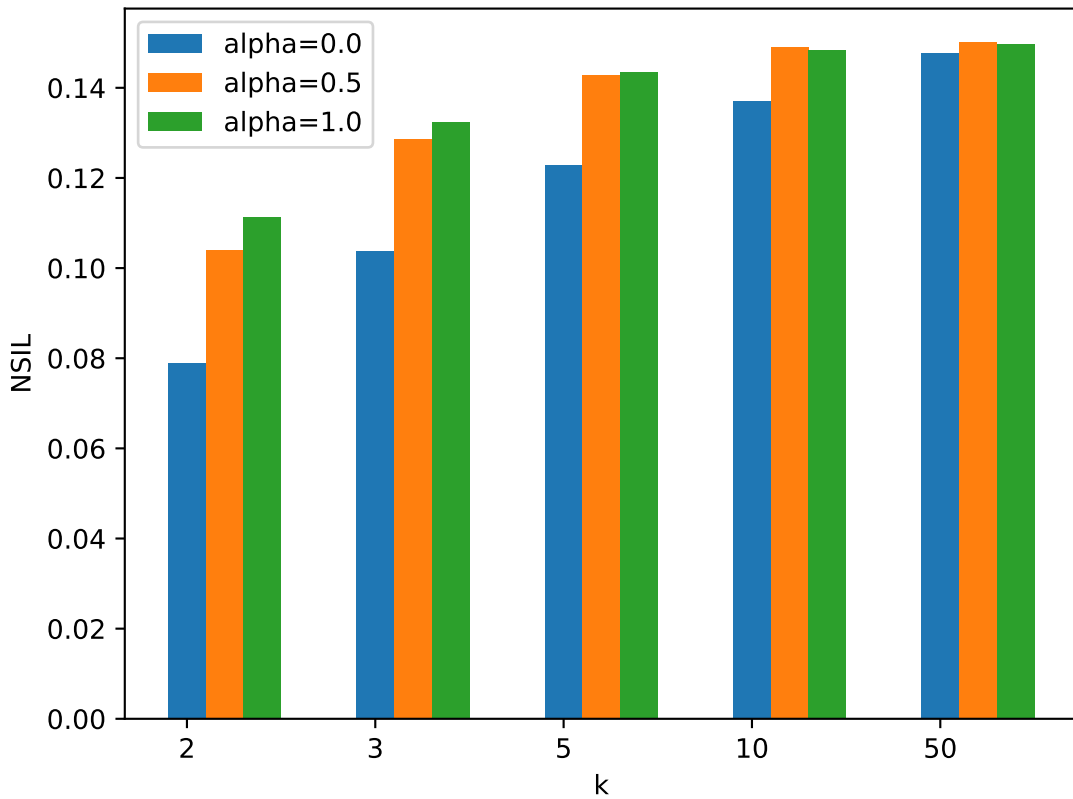
NSIL p=0.95
