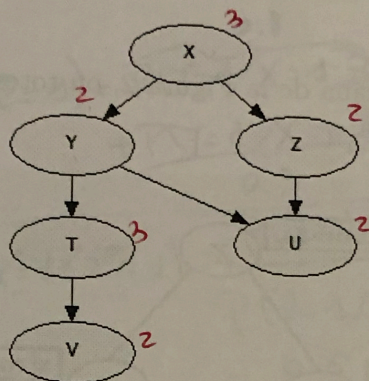
Figura 1: DAG Problema 1.
