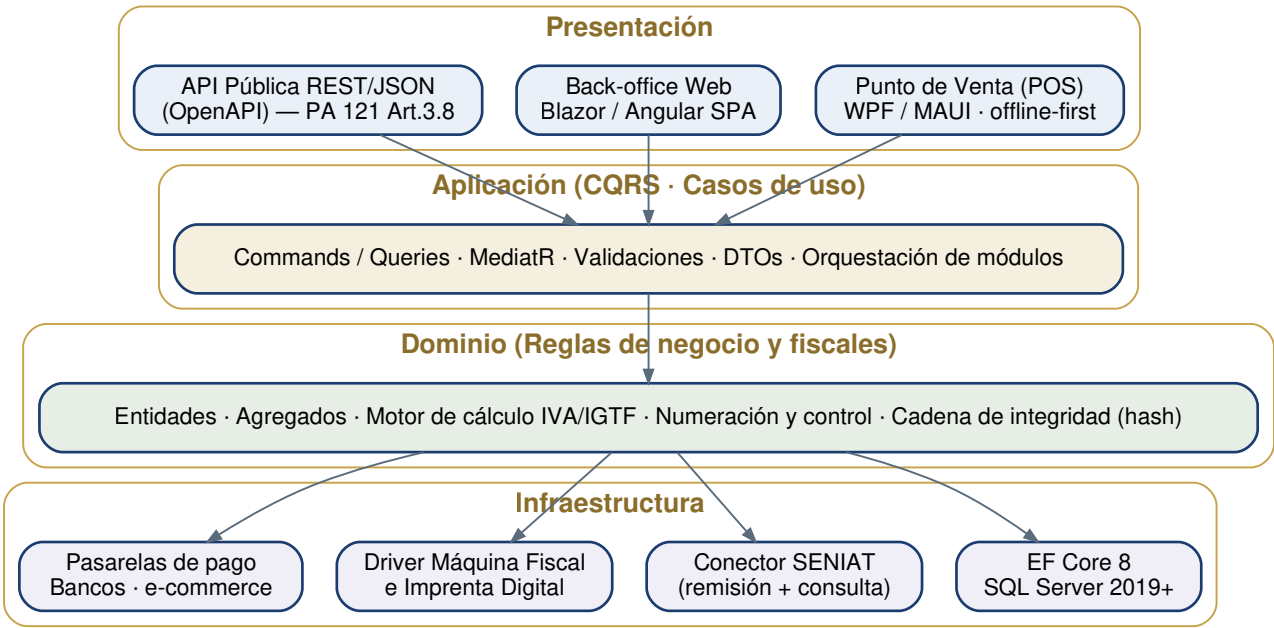
Figura 1. Arquitectura en capas (Clean Architecture) con el núcleo de dominio fiscal aislado.
