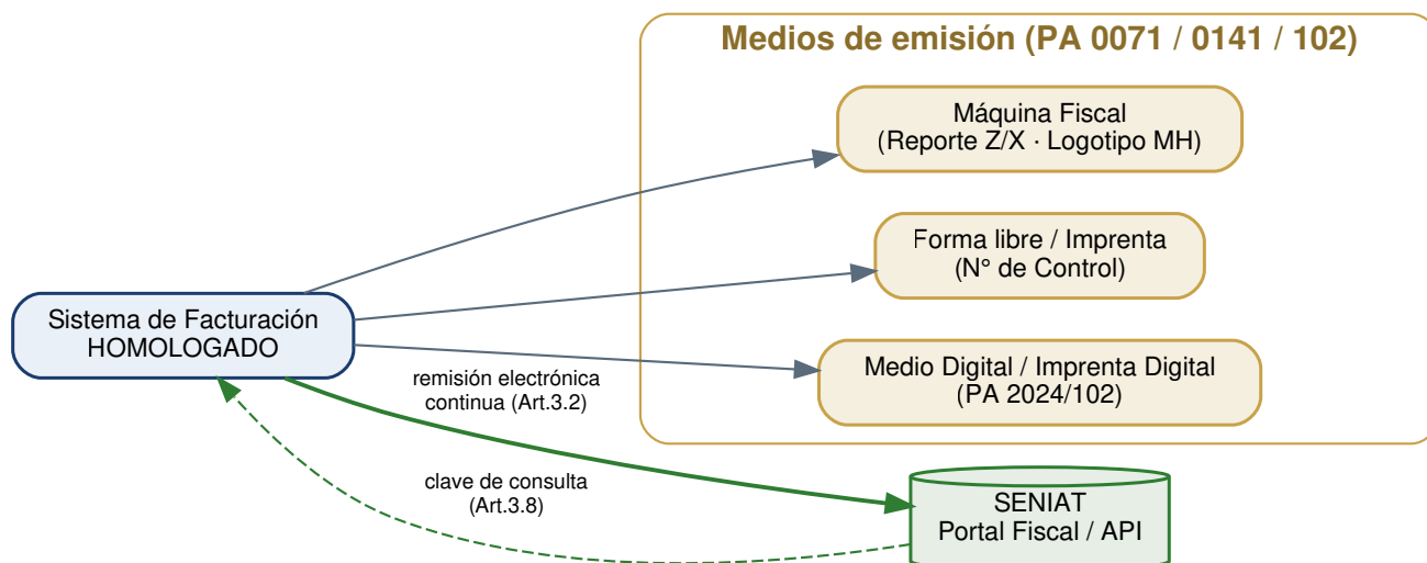
Figura 5. El sistema homologado orquesta los tres medios de emisión y mantiene el canal bidireccional con el SENIAT.
