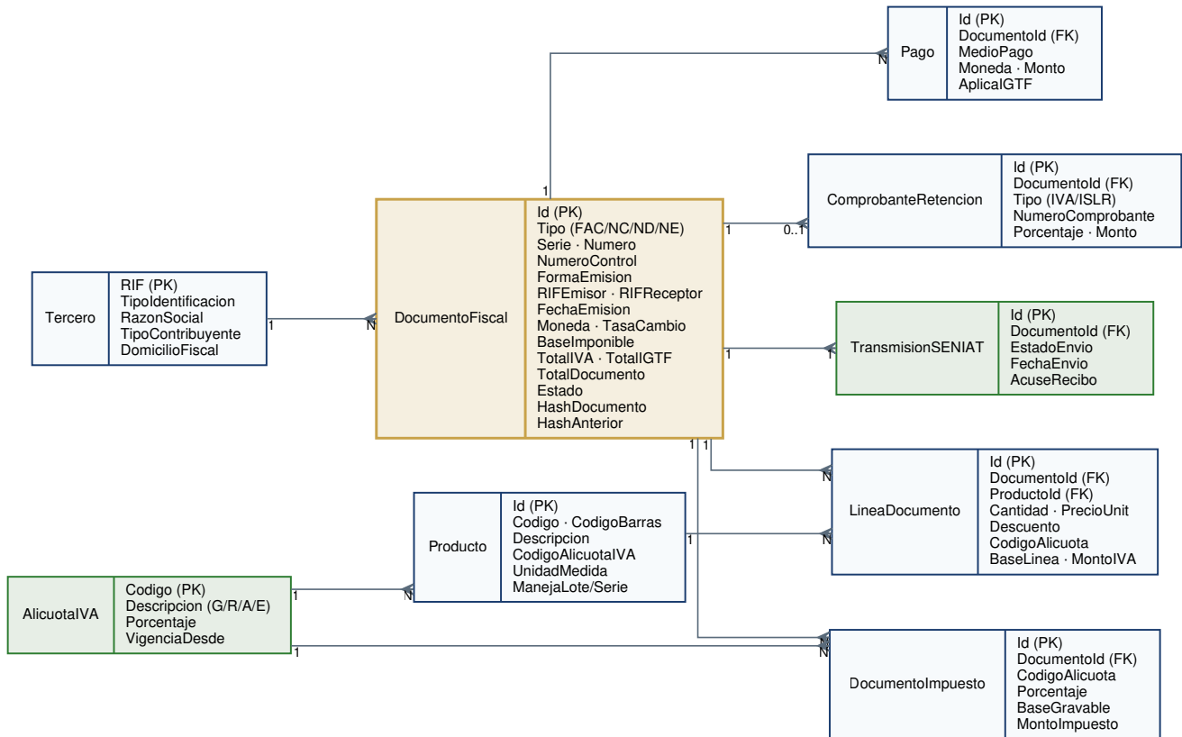
Figura 3. Modelo E-R del núcleo de facturación (M4/M6). En dorado el agregado raíz DocumentoFiscal; en verde las entidades de cumplimiento.
