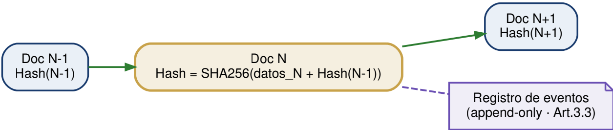
Figura 4. Cadena de integridad: cada documento incorpora el hash del anterior; el registro de eventos complementa la inviolabilidad.
