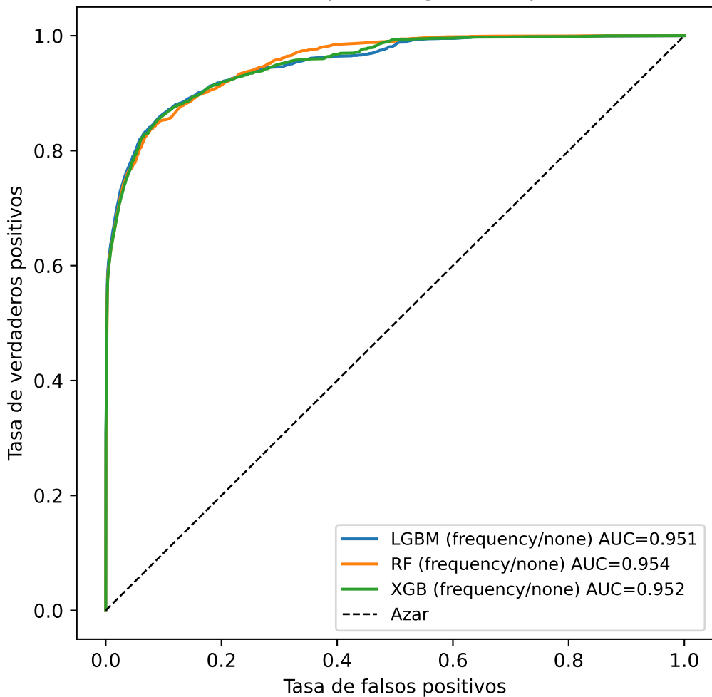
Curva ROC — mejor configuración por modelo
