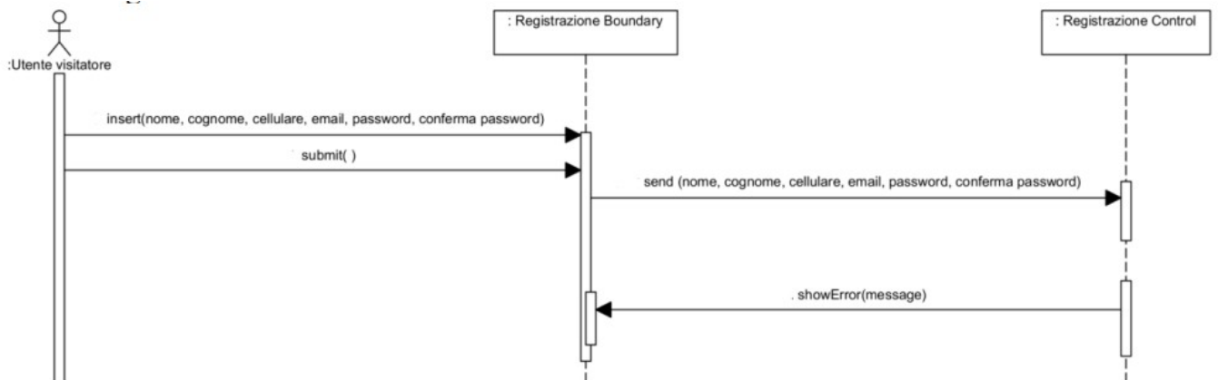
SD 1.1: Registrazione Utente Fallita
