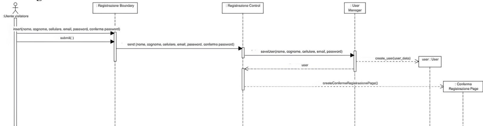
SD 1: Registrazione
