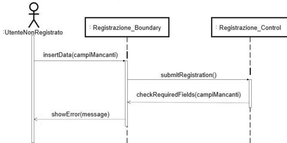
SD 1.2: Dati Mancanti Registrazione
