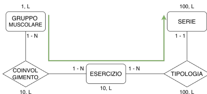
Figura 3.8: Schema di navigazione: Analisi volumetrica per gruppo muscolare
