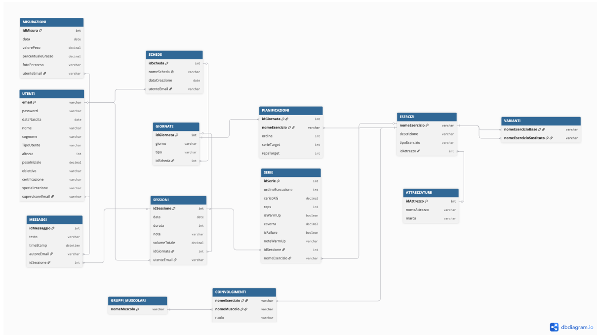
Figura 3.14: Schema relazionale finale con chiavi primarie e vincoli di integrità referenziale
