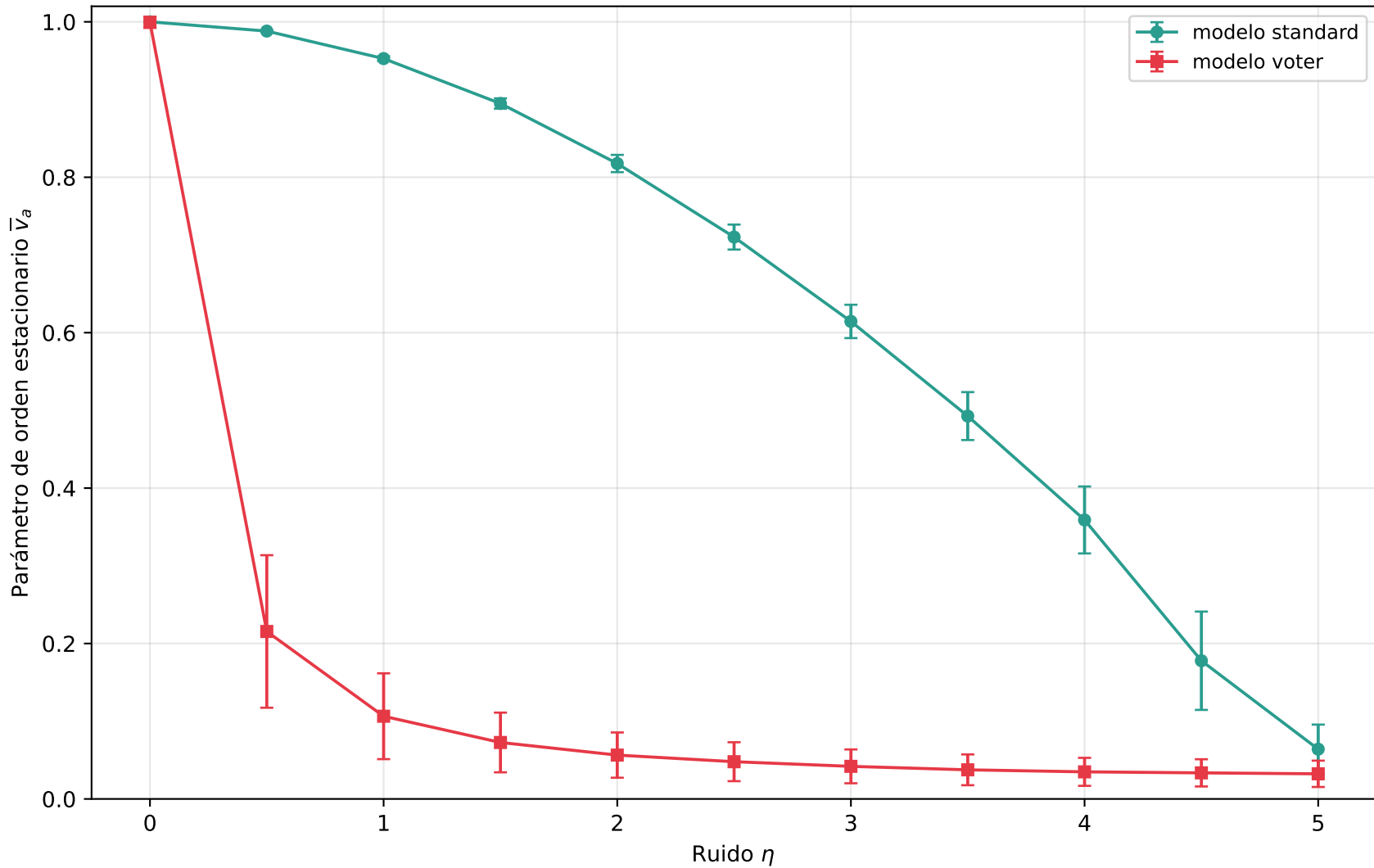
Parámetro de orden estacionario vs. ruido (transitorio descartado: 40%)
