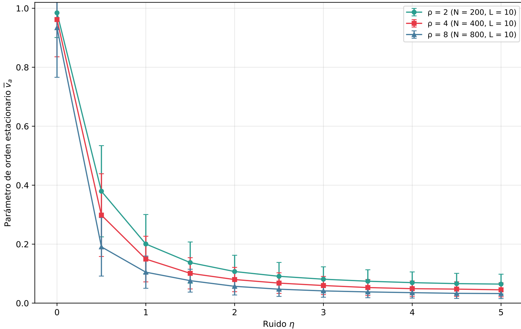
Parámetro de orden estacionario vs. ruido (transitorio descartado: 500)
