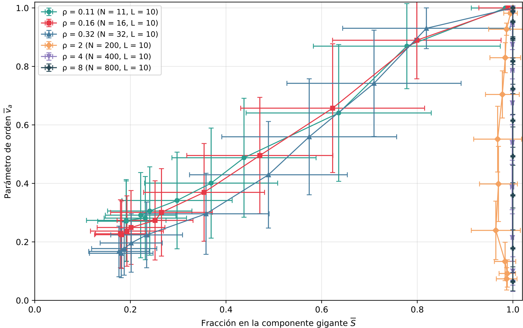
Polarización vs. componente gigante (promedios para t \geq 40\% )
