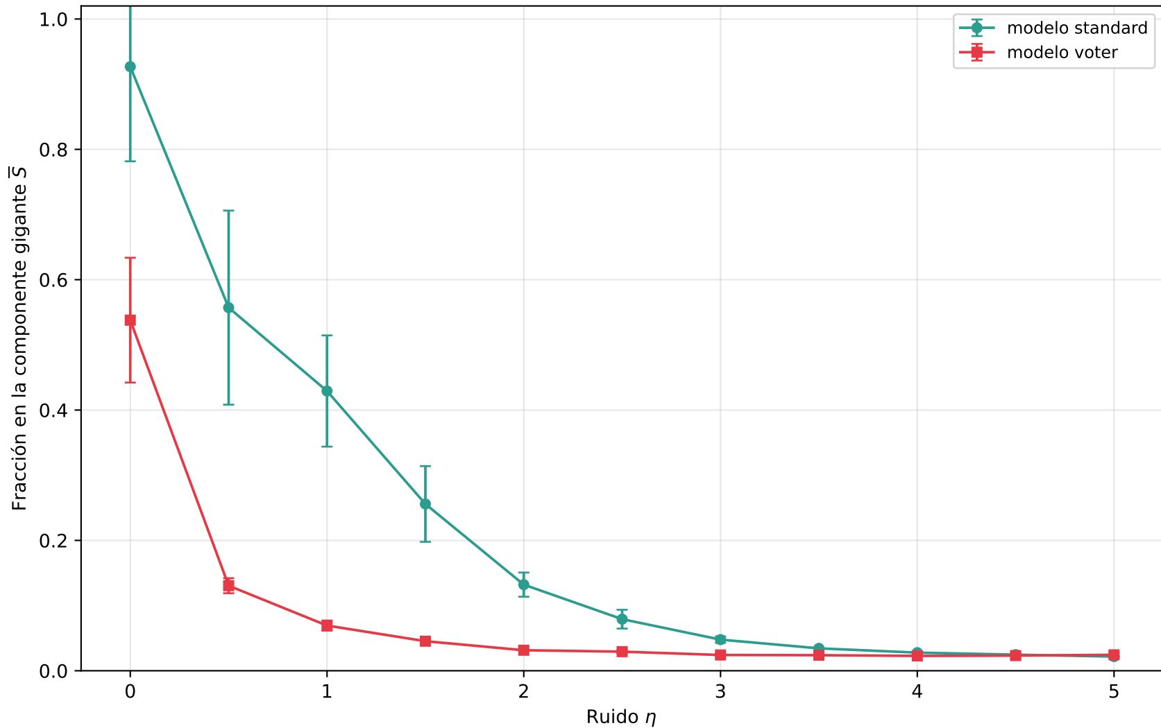
Componente gigante: estándar vs. votante ( \rho = 1/\pi )
