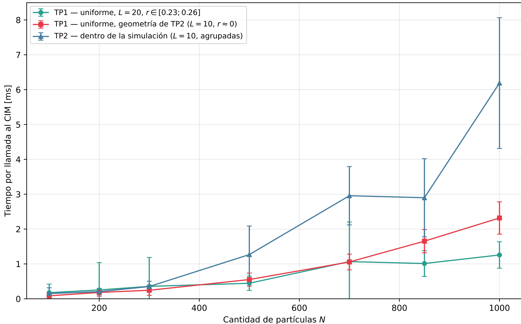
Tiempo del Cell Index Method: TP1 vs. TP2 ( r_c = 1 , periódico)
