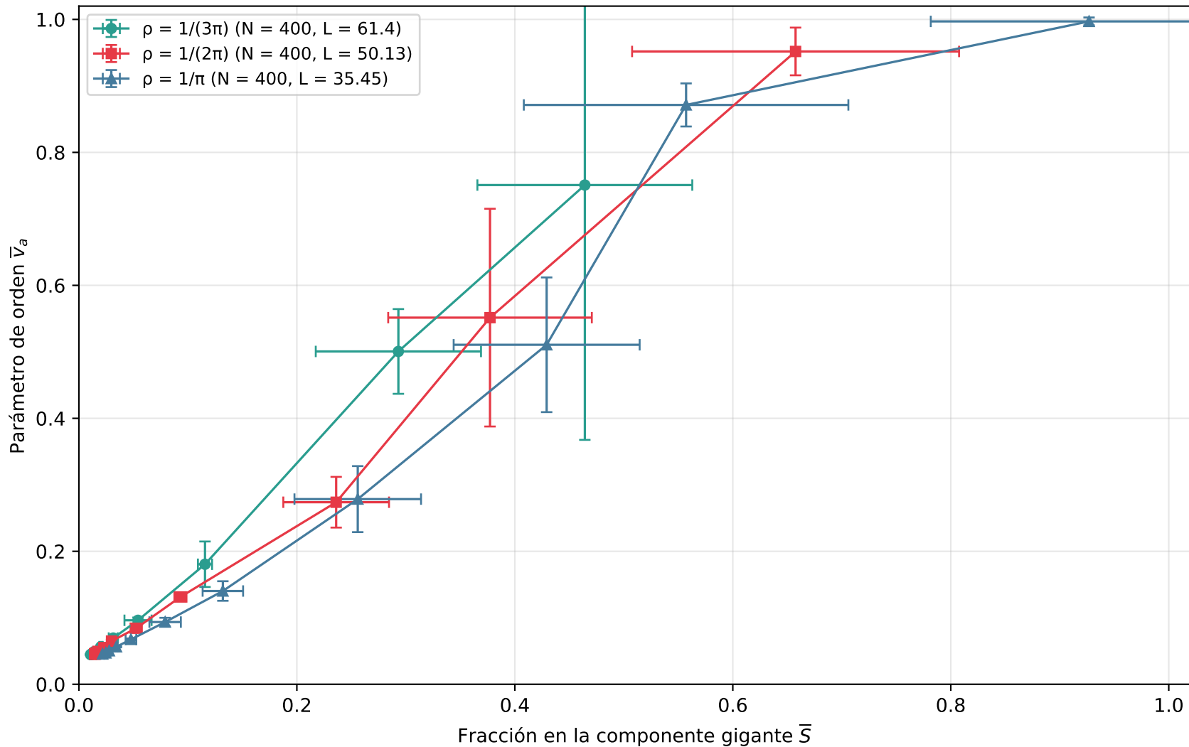
Polarización vs. componente gigante — densidades bajas ( N = 400 , T = 10000 )
