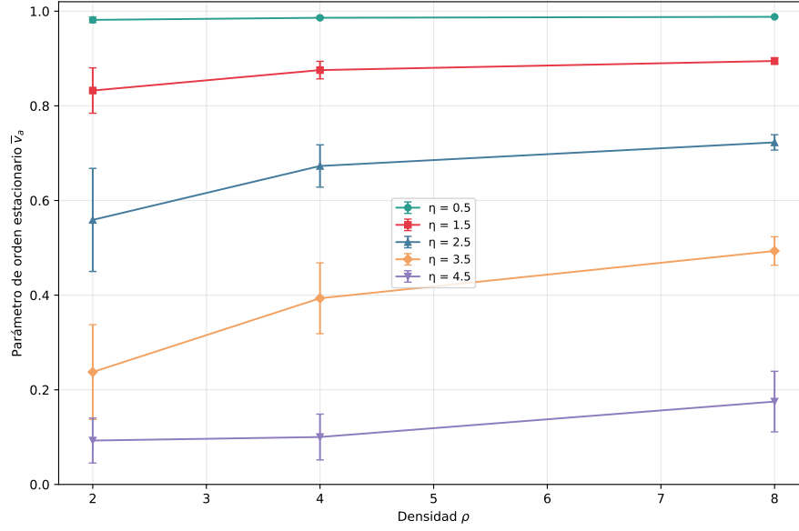
Figura 6: Parámetro de orden estacionario \langle \overline{v}_a \rangle en función de la densidad \rho , modelo estándar, para \eta = 0.5, 1.5, 2.5, 3.5, 4.5 (mismos datos de la Figura 5, transpuestos).
