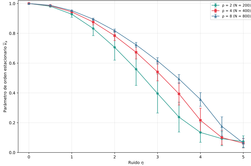
Figura 5: Polarización \langle v_a \rangle en función de \eta , modelo estándar, para \rho = 2, 4, 8 .
