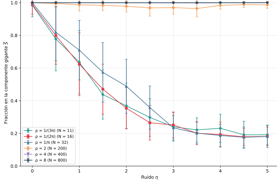
Figura 13: Tamaño relativo del cluster más grande \langle \bar{S} \rangle en función de \eta , para \rho = 2, 4, 8, \frac{1}{\pi}, \frac{1}{2\pi}, \frac{1}{3\pi} .
