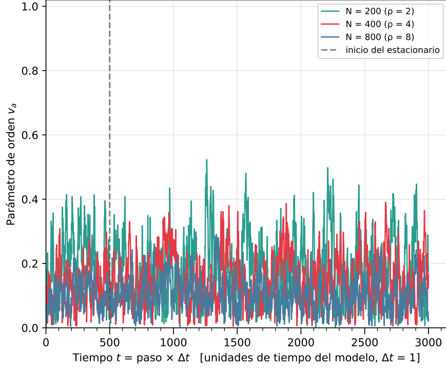
Figura 8: Evolución temporal de la polarización v_a(t) para una corrida representativa con \eta = 1 , modelo votante, para \rho = 2, 4, 8 . La línea vertical en t = 500 marca el corte usado para descartar el transitorio al promediar el estado estacionario.
