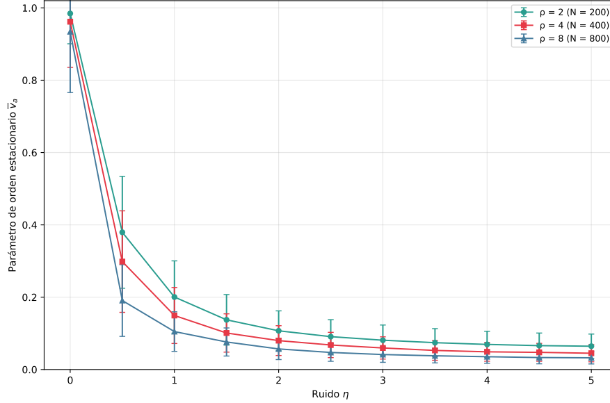
Figura 9: Polarización \langle v_a \rangle en función de \eta , modelo votante, para \rho = 2, 4, 8 .
