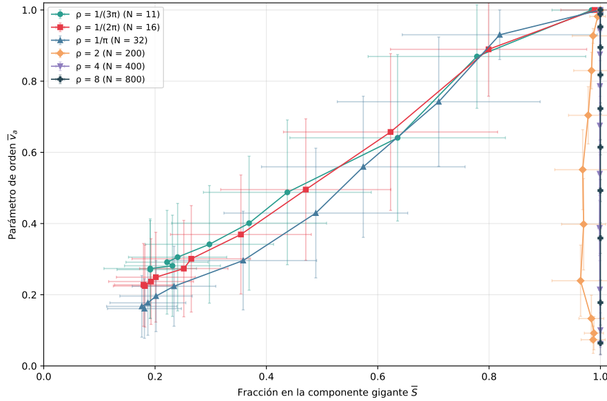
Figura 14: Relación entre la polarización \bar{v}_a y el tamaño de cluster \bar{S} .
