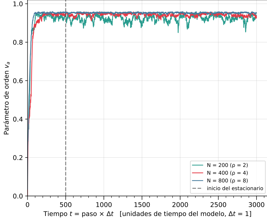
Figura 4: Evolución temporal de la polarización v_a(t) para una corrida representativa con \eta = 1 , modelo estándar, para \rho = 2, 4, 8 . La línea vertical en t = 500 marca el corte usado para descartar el transitorio al promediar el estado estacionario.
