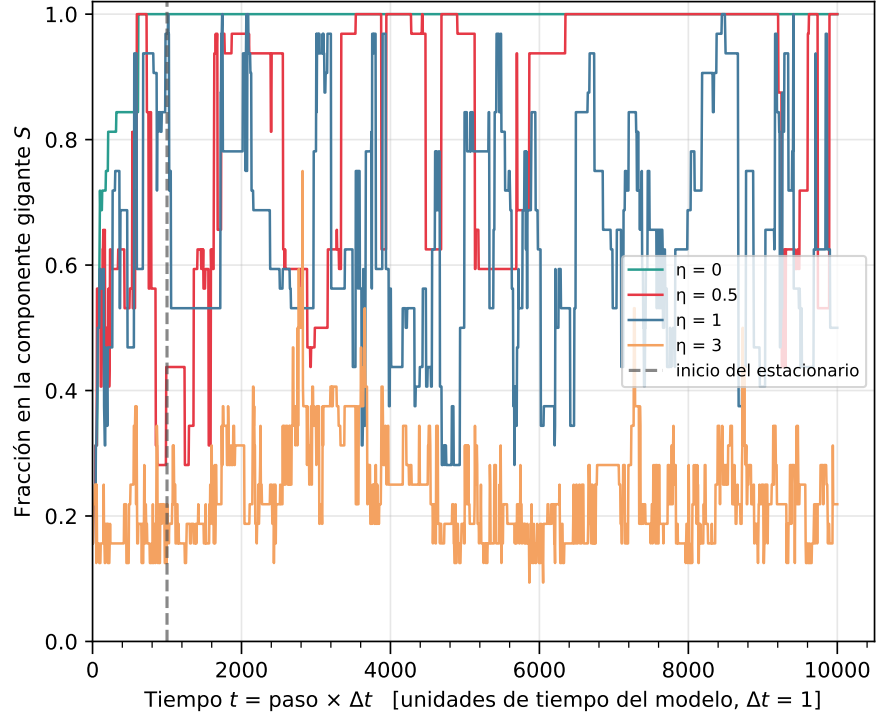
Figura 10: Evolución temporal de la fracción en la componente gigante S(t) para \rho = 1/\pi ( N = 32 , L = 10 ), modelo estándar, con \eta = 0, 0.5, 1, 3 . La línea vertical en t = 1000 marca el corte usado para descartar el transitorio al promediar el estado estacionario.
