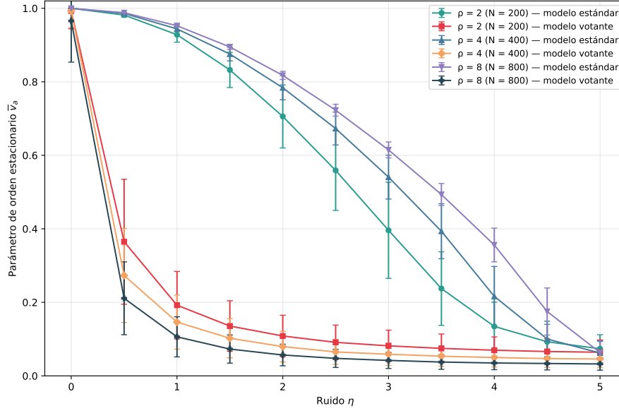
Figura 15: Comparación entre el modelo estándar y el modelo votante, para \rho = 2, 4, 8 .
