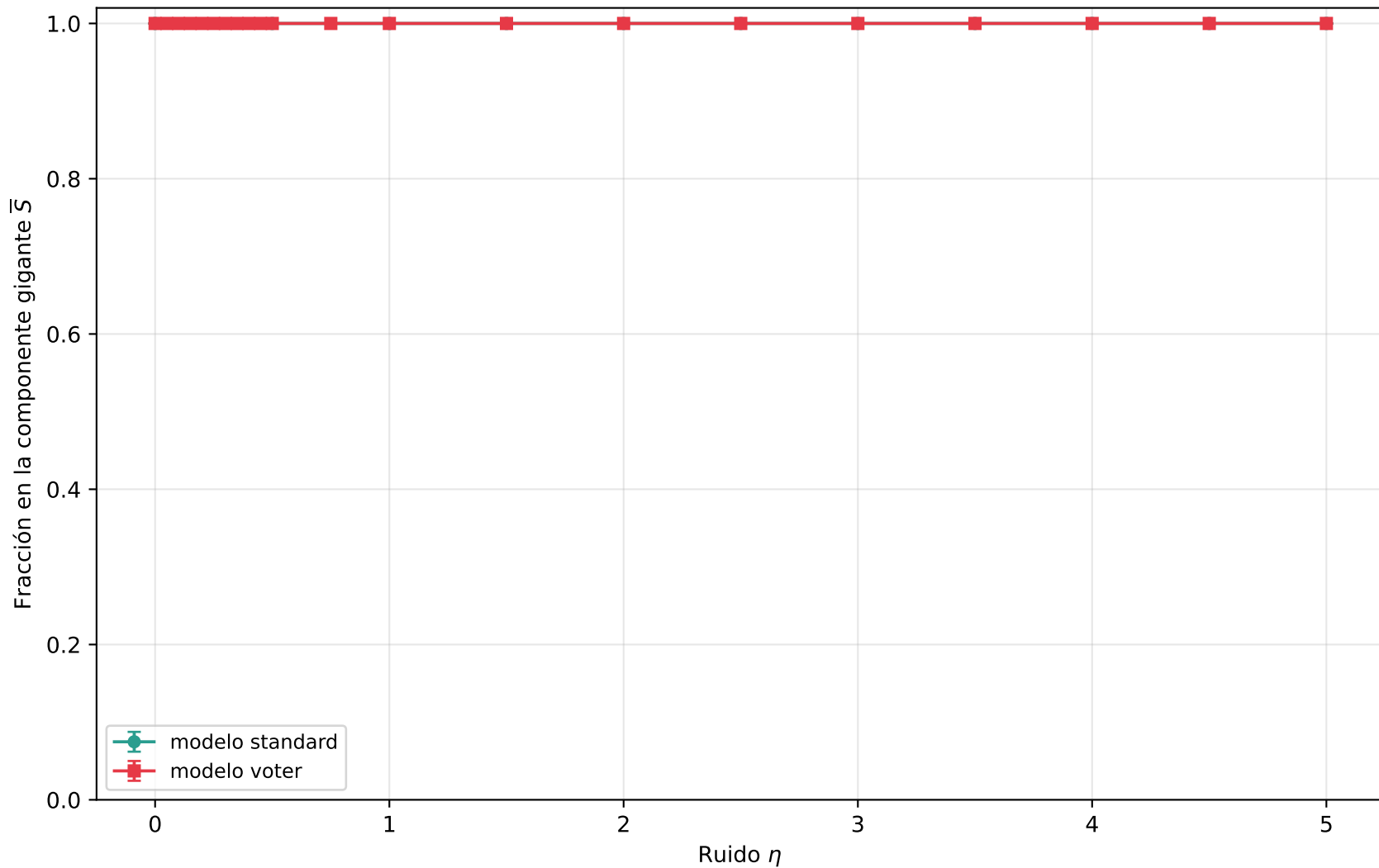
Componente gigante: estándar vs. votante ( \rho = 8 )
