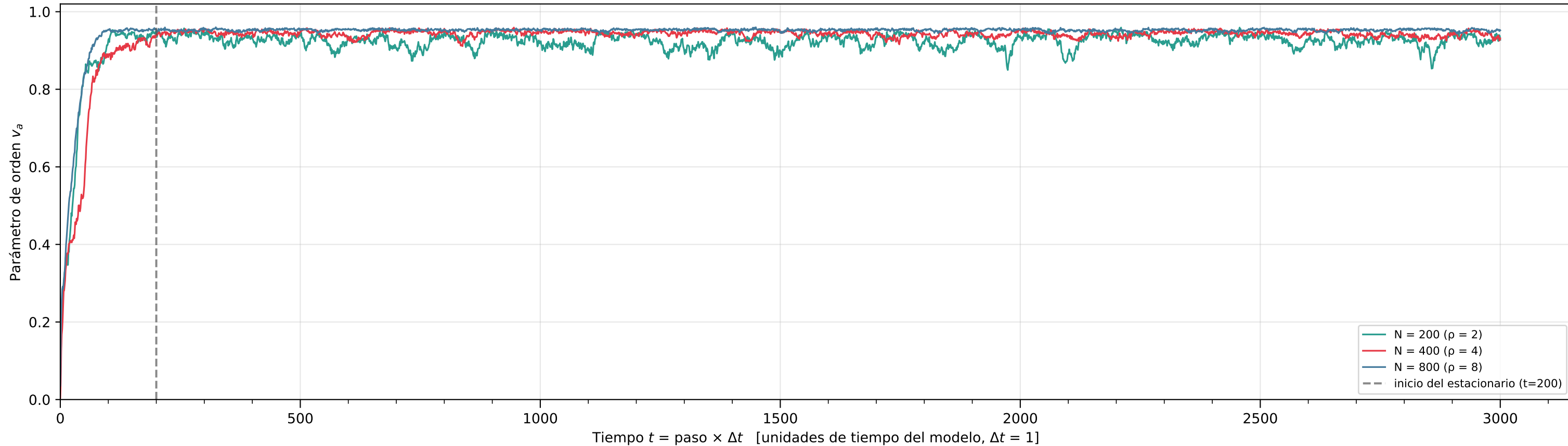
Evolución temporal de v_a — modelo estándar ( \theta_0 aleatorio, \eta = 1 , L = 10 )
