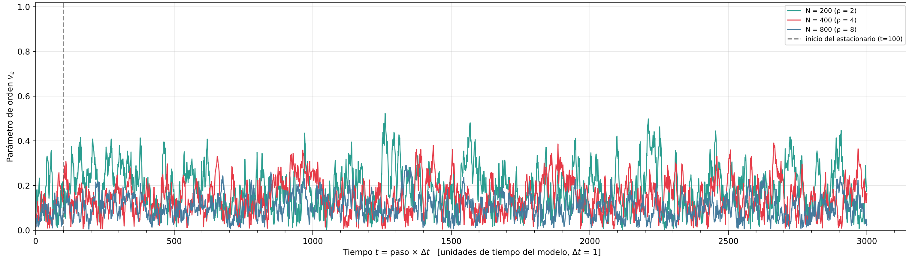
Evolución temporal de v_a — modelo votante ( \theta_0 aleatorio, \eta = 1 , L = 10 )
