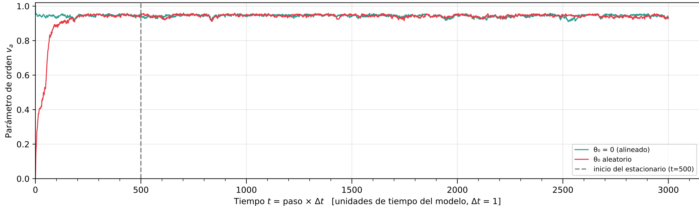
Parámetro de orden v_a vs. tiempo — Modelo standard, N=400 , \rho=4 , \eta=1
