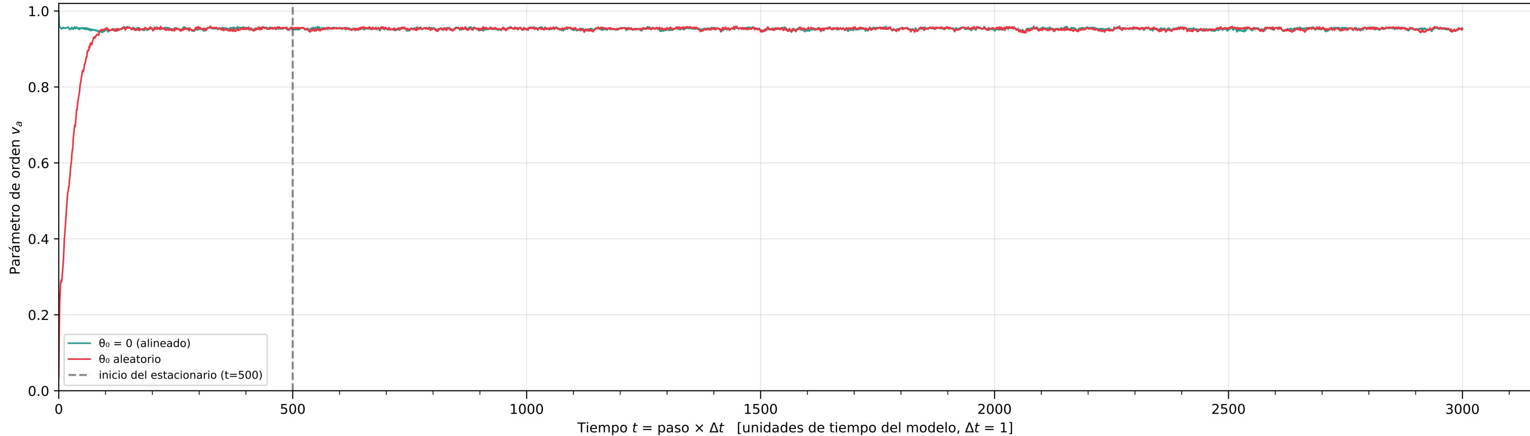
Criterio de estacionario — modelo estándar, \rho = 8 , \eta = 1
