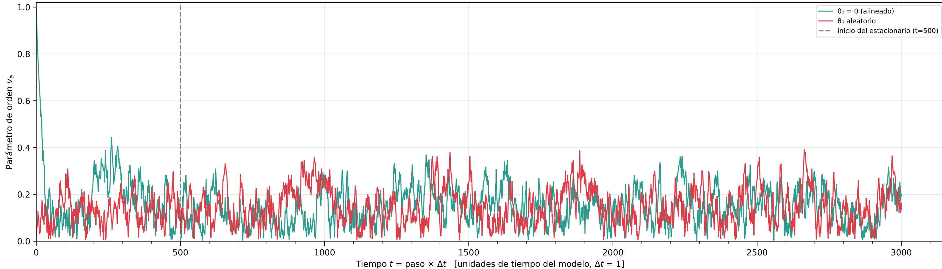
Criterio de estacionario — modelo votante, \rho = 4 , \eta = 1
