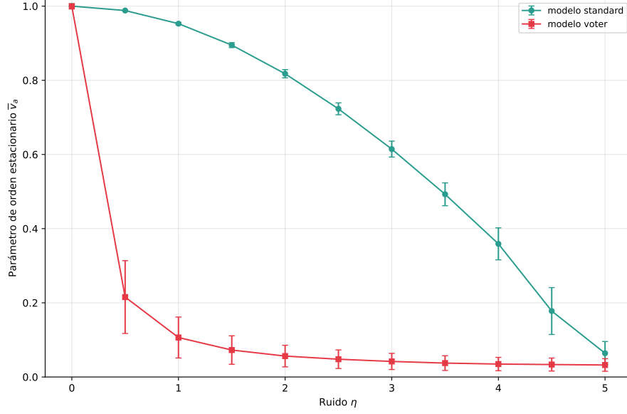
Figura 10: Comparación entre el modelo estándar y el modelo votante, \rho = 8 .
