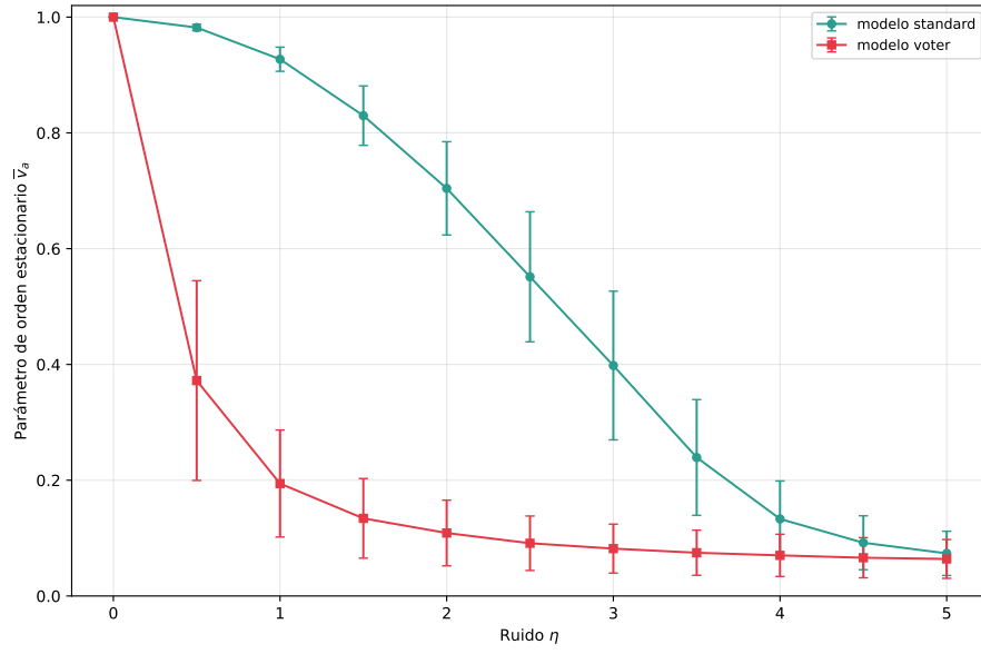
Figura 8: Comparación entre el modelo estándar y el modelo votante, \rho = 2 .
