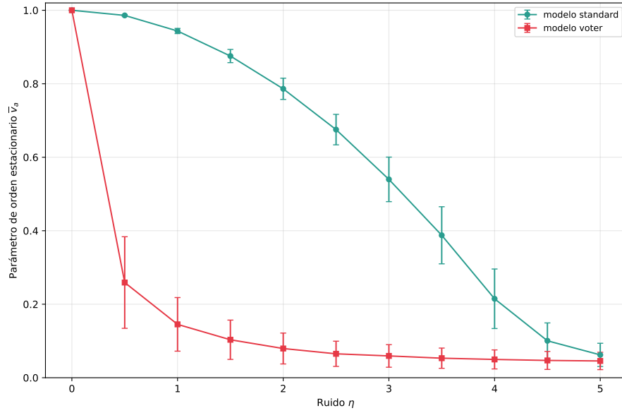
Figura 9: Comparación entre el modelo estándar y el modelo votante, \rho = 4 .
