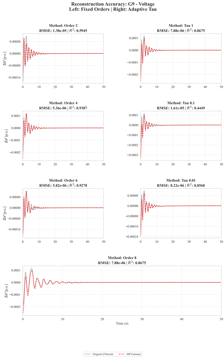
Σχήμα Α'52: Ανακατασκευή σήματος τάσης ( V ) για τη γεννήτρια G_9 του IEEE 39-Bus System.
