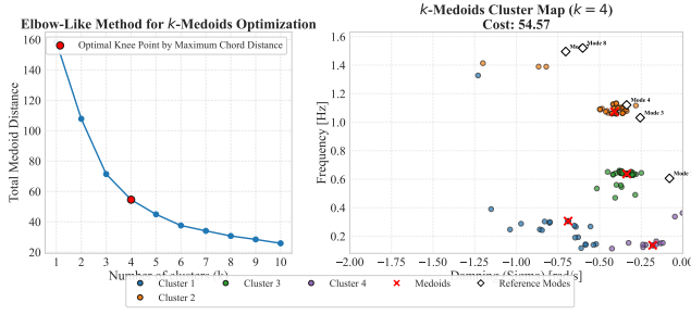
Fig. 27. Διάγραμμα Elbow του αλγορίθμου k -Medoids για την περιοχή ελέγχου 3 του IEEE 39-Bus System .
