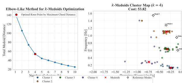
Fig. 25. Διάγραμμα Elbow του αλγορίθμου k -Medoids για την περιοχή ελέγχου 1 του IEEE 39-Bus System .
