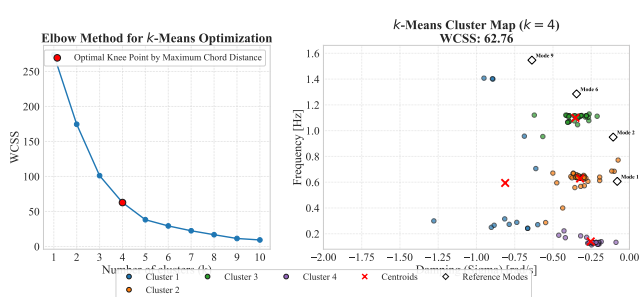
Fig. 19. Διάγραμμα Elbow του αλγορίθμου k -Means για την περιοχή ελέγχου 1 του IEEE 39-Bus System .
