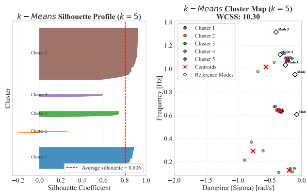
Fig. 23. Silhouette profile του αλγορίθμου k -Means για k = 5 στην περιοχή ελέγχου 2 του IEEE 39-Bus System .
