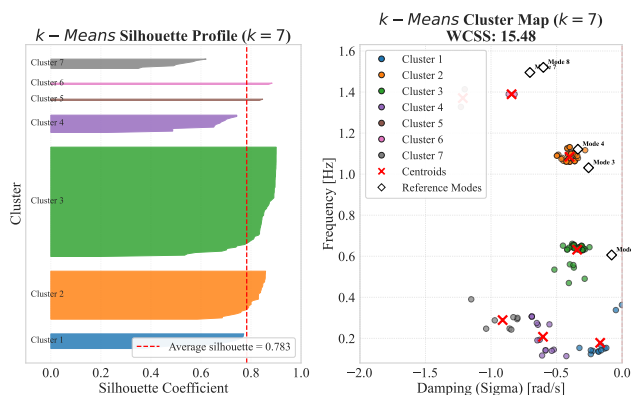
Fig. 24. Silhouette profile του αλγορίθμου k -Means για k = 7 στην περιοχή ελέγχου 3 του IEEE 39-Bus System .
