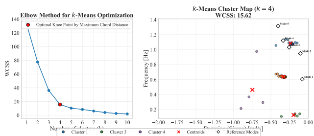
Fig. 20. Διάγραμμα Elbow του αλγορίθμου k -Means για την περιοχή ελέγχου 2 του IEEE 39-Bus System .
