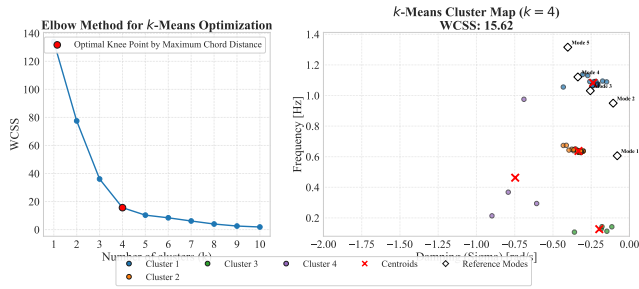
Fig. 20. Διάγραμμα Elbow του αλγορίθμου k -Means για την περιοχή ελέγχου 2 του IEEE 39-Bus System .
