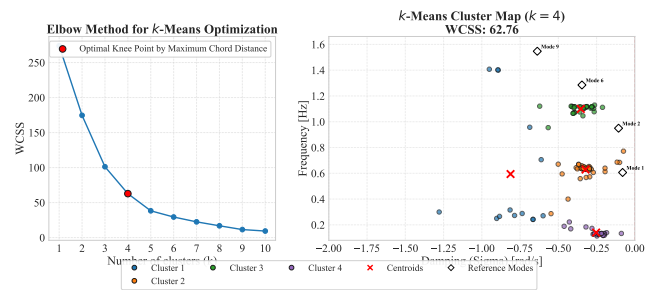
Fig. 19. Διάγραμμα Elbow του αλγορίθμου k -Means για την περιοχή ελέγχου 1 του IEEE 39-Bus System.
