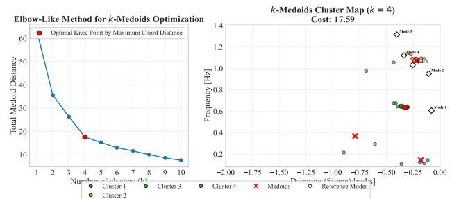
Fig. 26. Διάγραμμα Elbow του αλγορίθμου k -Medoids για την περιοχή ελέγχου 2 του IEEE 39-Bus System .
