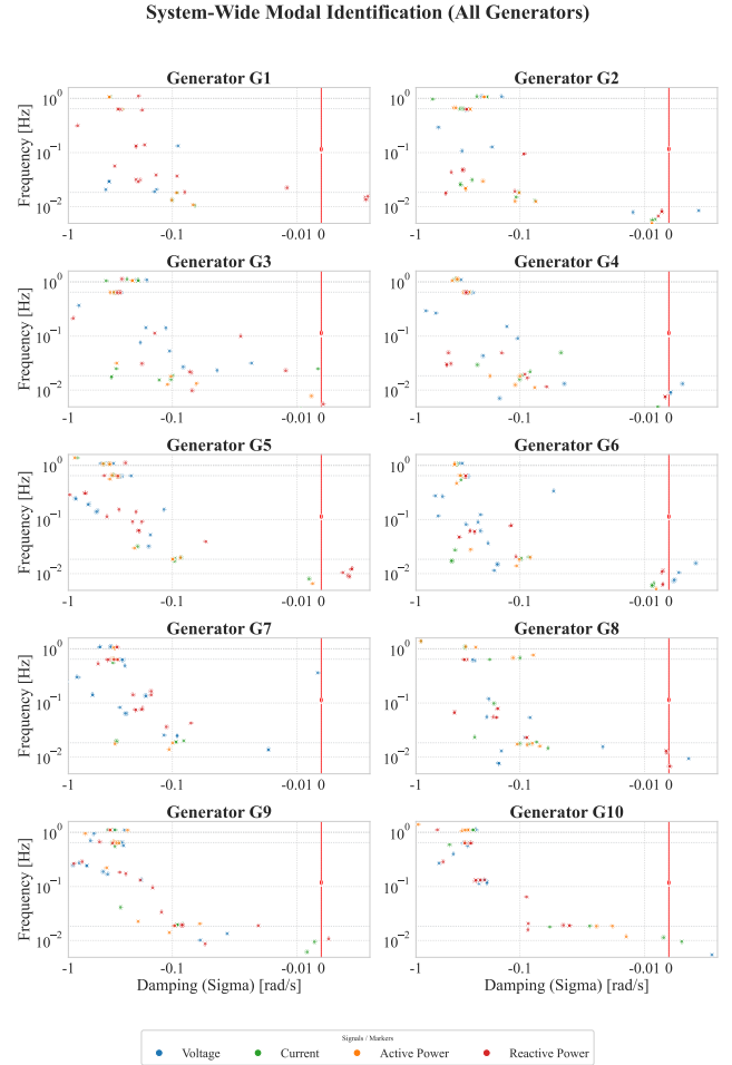
Fig. 2. Κατανομή ιδιοτιμών (Real Part vs Frequency) για τις γεννήτριες G_1 - G_{10} του IEEE 39-Bus System .
