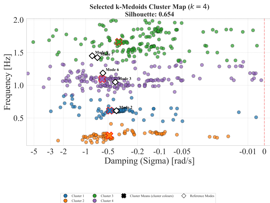
Σχήμα 4.3: Selected cluster map για το πρώτο order sweep και την Περιοχή 3: k-Medoids.
