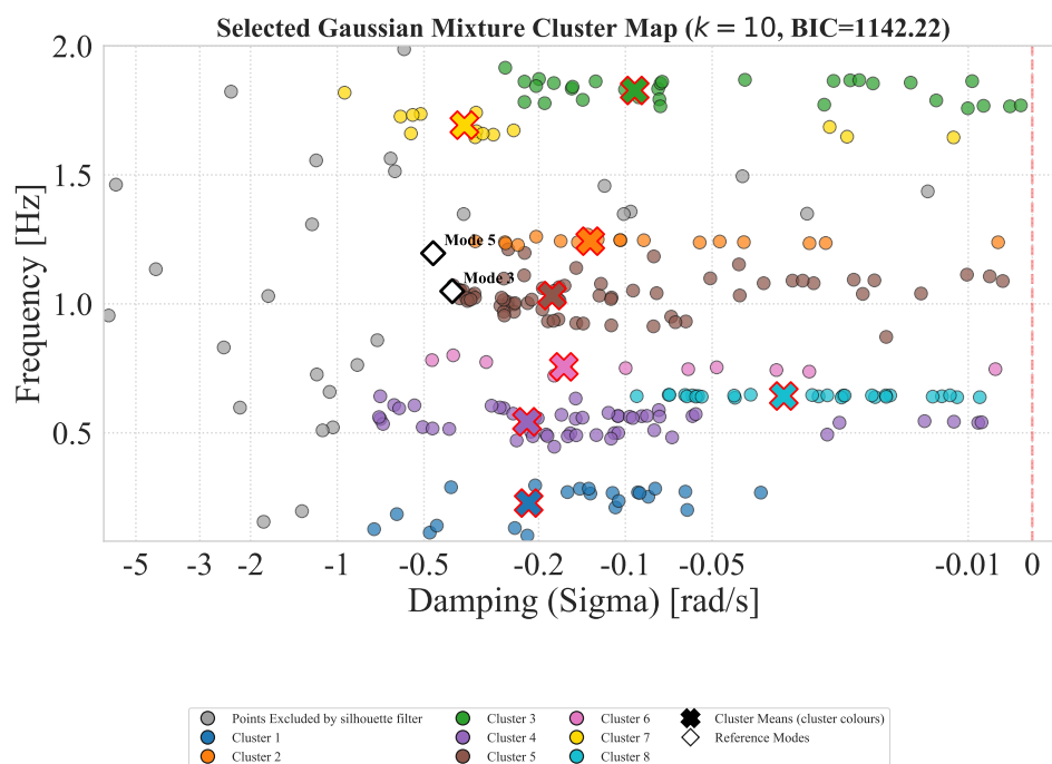
Σχήμα Β'.34: Selected cluster map: GMM (orders2).
