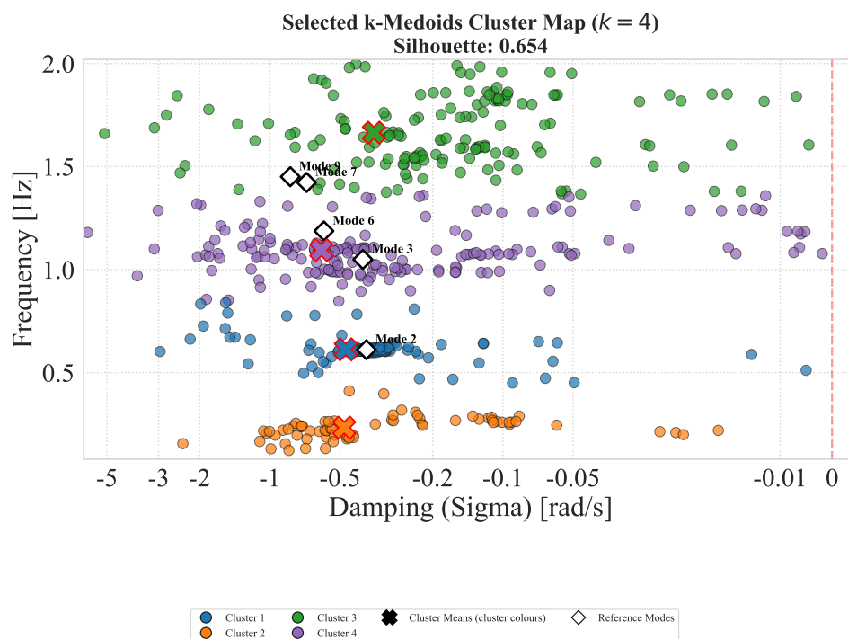
Σχήμα Β'.16: Selected cluster map: k-Medoids (orders1).
