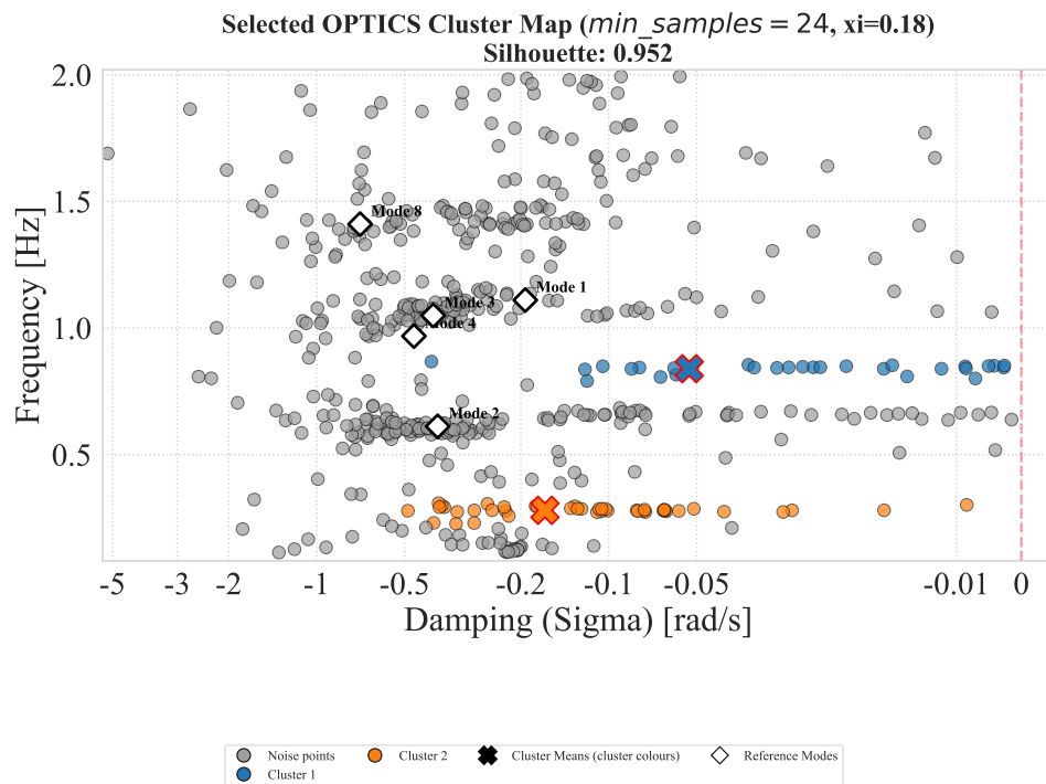
Σχήμα Β'.4: Selected cluster map: OPTICS (orders1).
