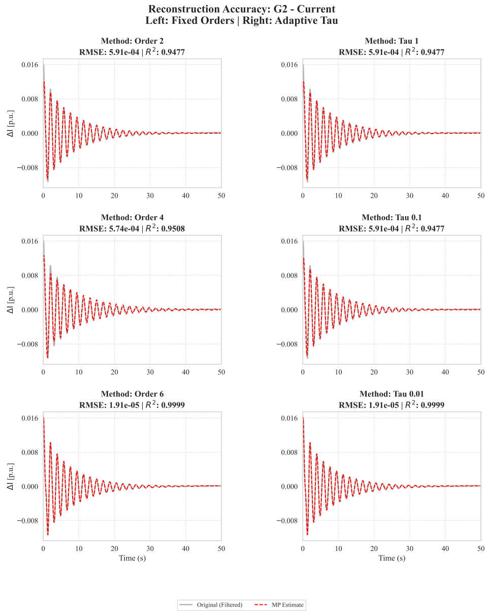
Σχήμα Α'.6: Ανακατασκευή σήματος ρεύματος ( I ) για τη γεννήτρια G_2 του Kundur Two-Area System.
