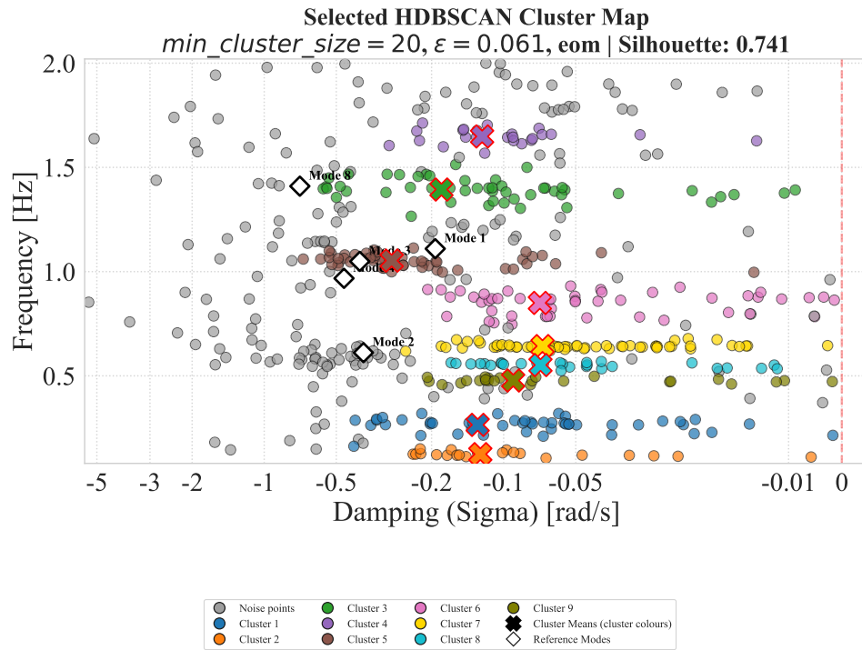
Σχήμα Β'.26: Selected cluster map: HDBSCAN (orders2).
