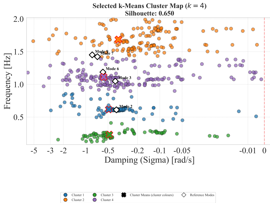
Σχήμα 4.2: Selected cluster map για το πρώτο order sweep και την Περιοχή 3: k-Means.
