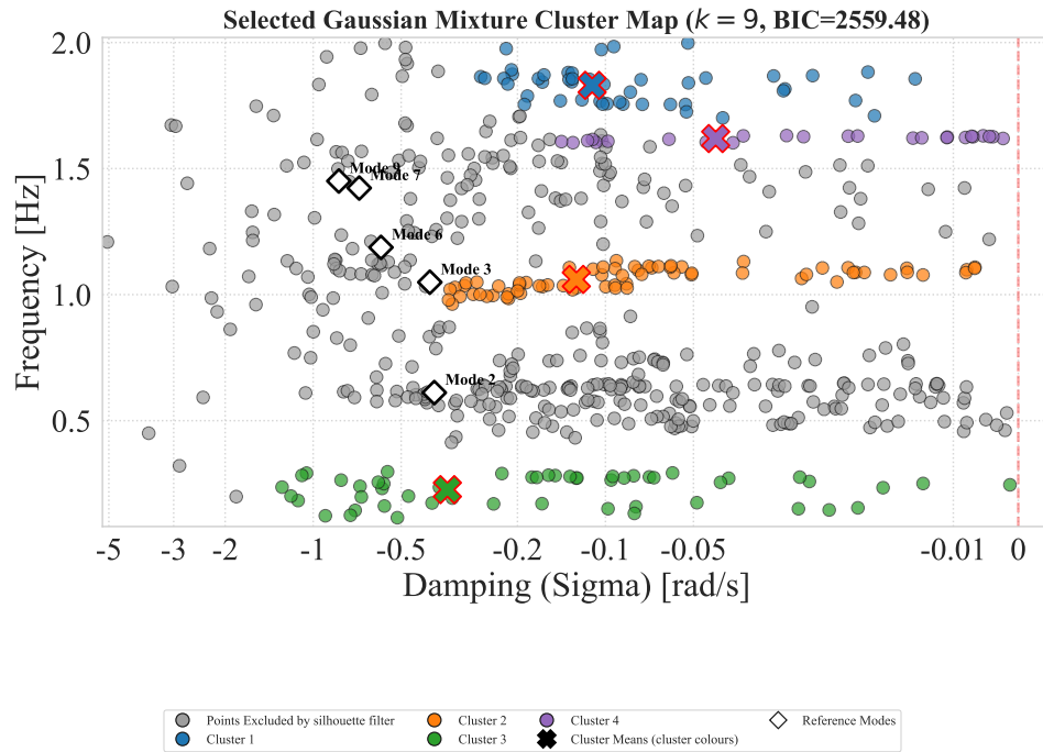
Σχήμα Β'.41: Selected cluster map: GMM (orders2).
