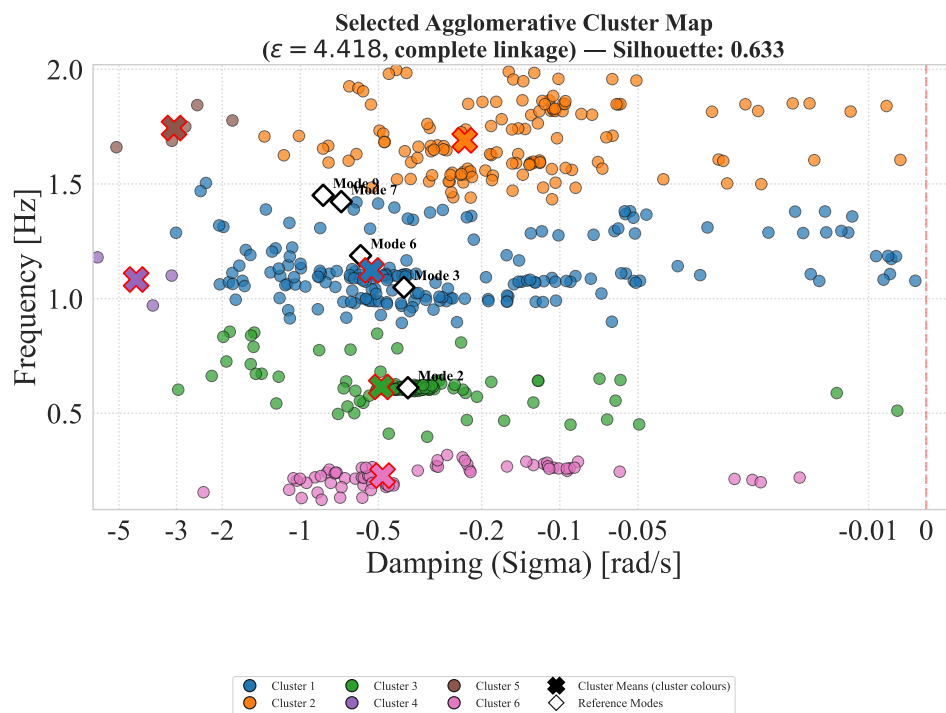
Σχήμα 4.8: Selected cluster map για το πρώτο order sweep και την Περιοχή 3: Agglomerative Hierarchical Clustering.
