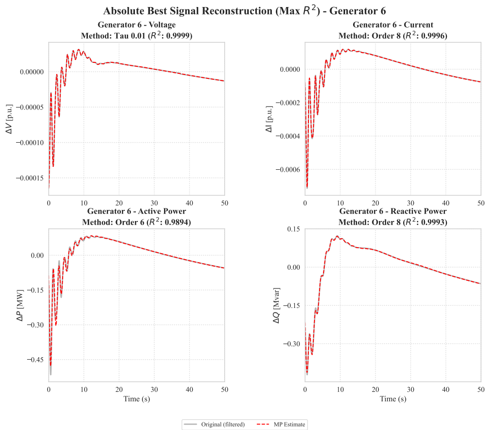
Σχήμα 3.11: Βέλτιστη μαθηματική ανακατασκευή των σημάτων ( V, I, P, Q ) για τη γεννήτρια G_6 του IEEE 39-Bus System με βάση τον μέγιστο συντελεστή προσδιορισμού R^2 .
