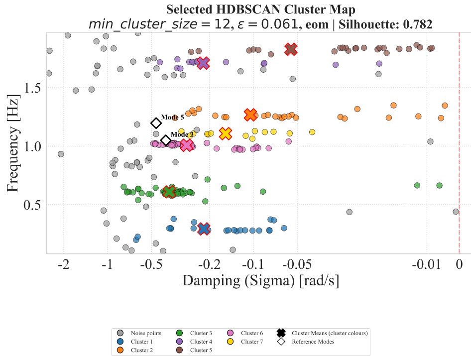
Σχήμα Β'.12: Selected cluster map: HDBSCAN (orders1).
