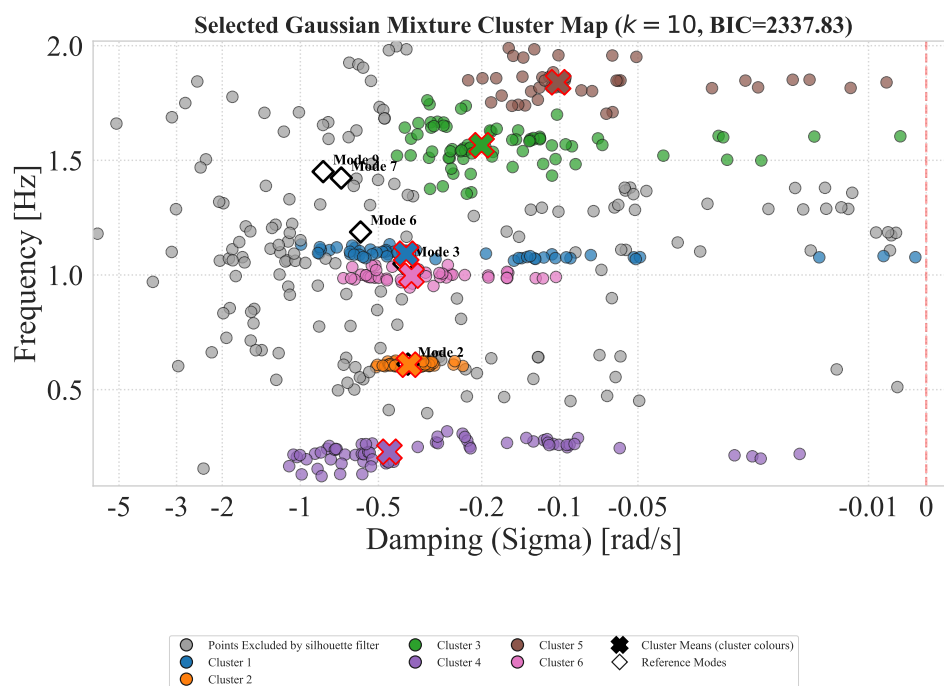
Σχήμα Β'.20: Selected cluster map: GMM (orders1).
