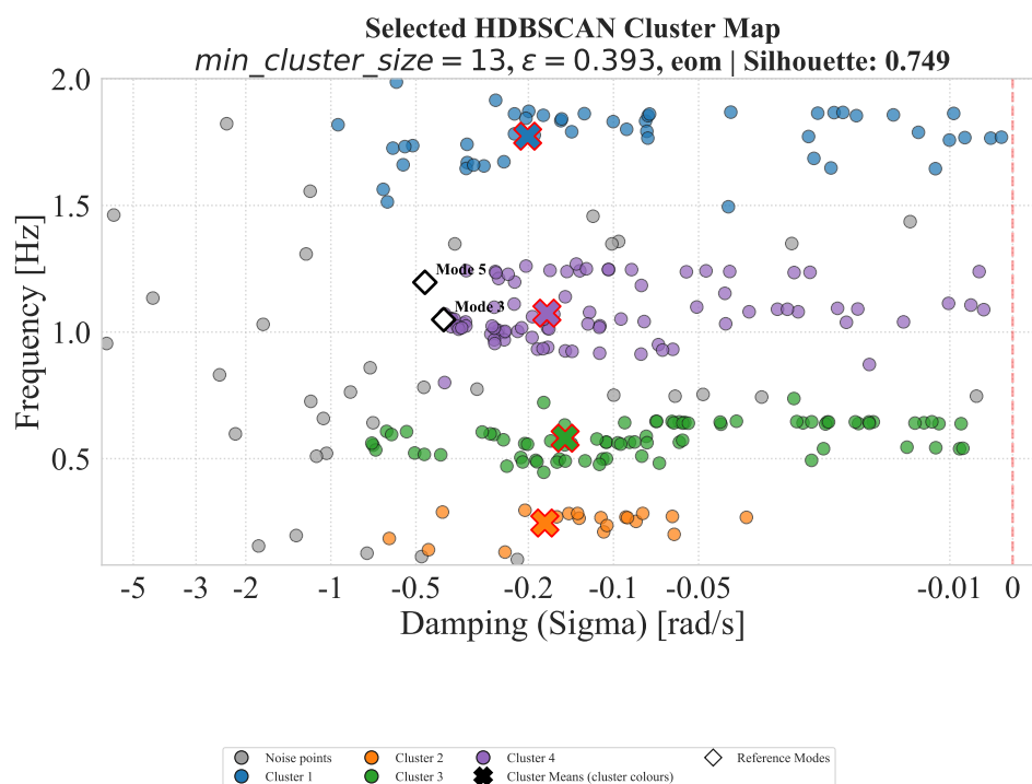
Σχήμα Β'.33: Selected cluster map: HDBSCAN (orders2).
