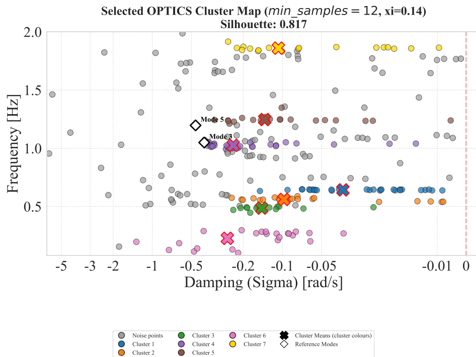
Σχήμα Β'.32: Selected cluster map: OPTICS (orders2).
