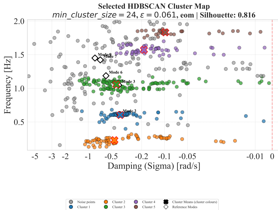
Σχήμα 4.4: Selected cluster map για το πρώτο order sweep και την Περιοχή 3: HDBSCAN.
