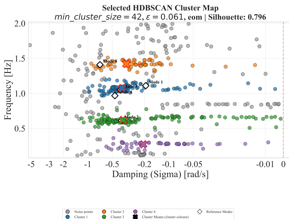
Σχήμα Β'.5: Selected cluster map: HDBSCAN (orders1).
