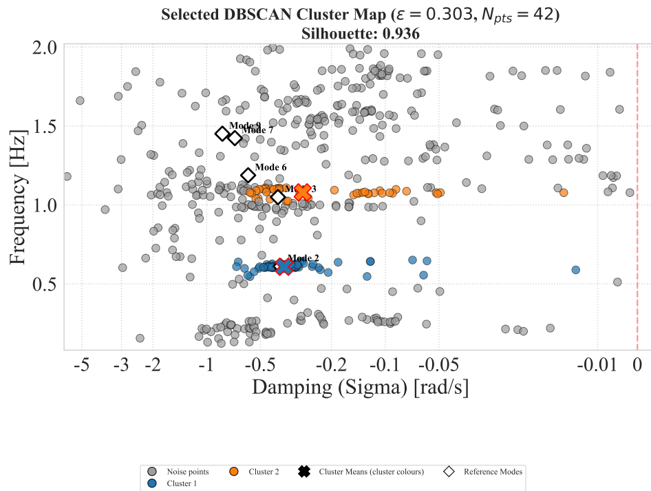
Σχήμα 4.6: Selected cluster map για το πρώτο order sweep και την Περιοχή 3: DBSCAN.
