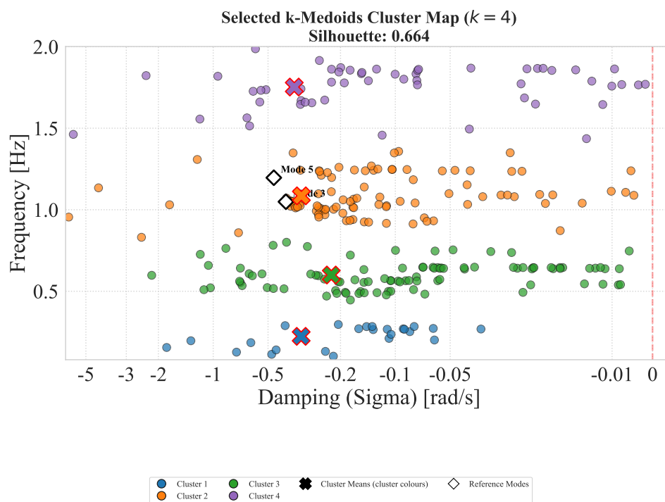
Σχήμα Β'.30: Selected cluster map: k -Medoids (orders2).
