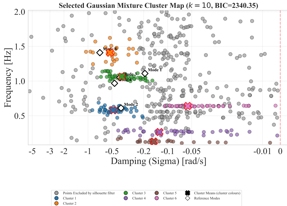
Σχήμα Β'.27: Selected cluster map: GMM (orders2).
