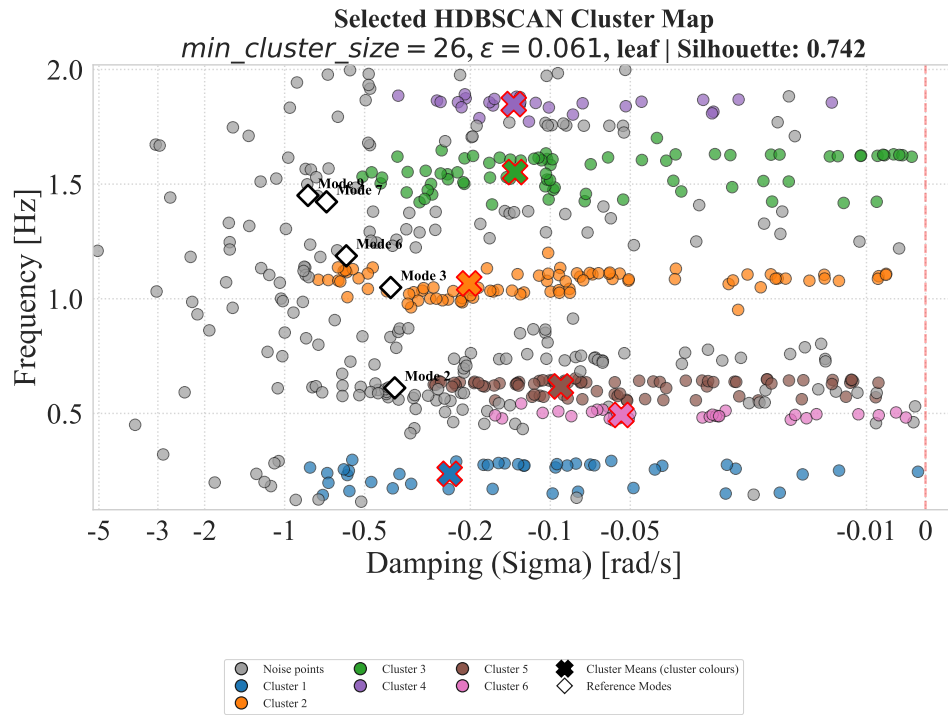
Σχήμα Β'.40: Selected cluster map: HDBSCAN (orders2).
