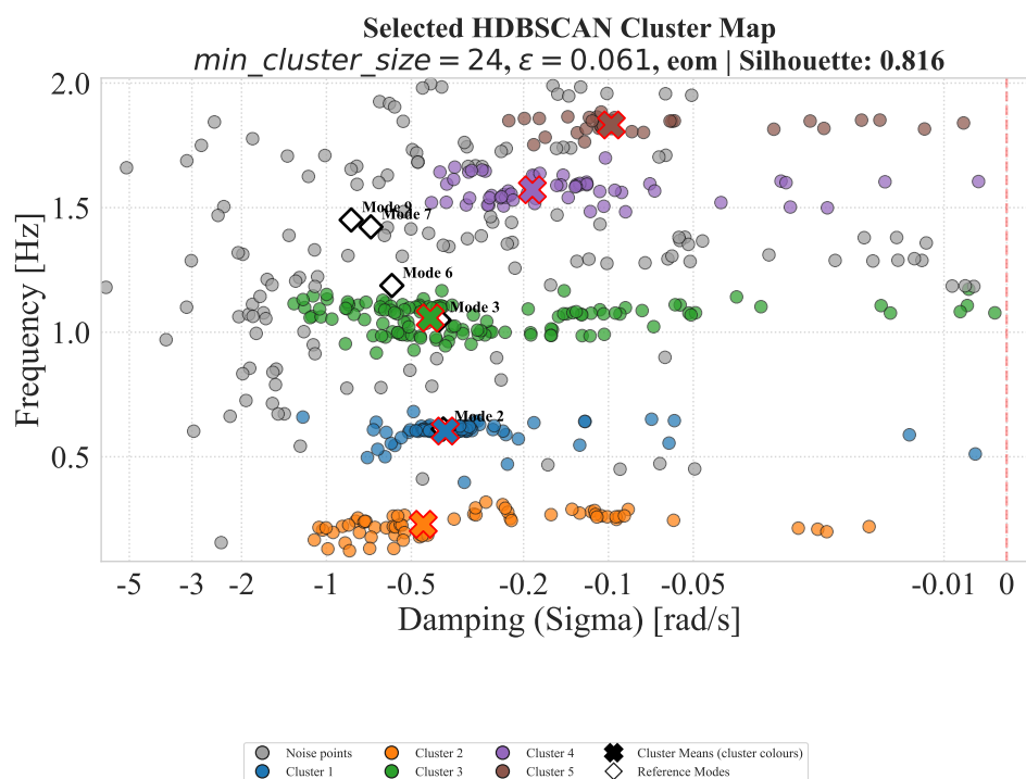
Σχήμα Β'.19: Selected cluster map: HDBSCAN (orders1).
