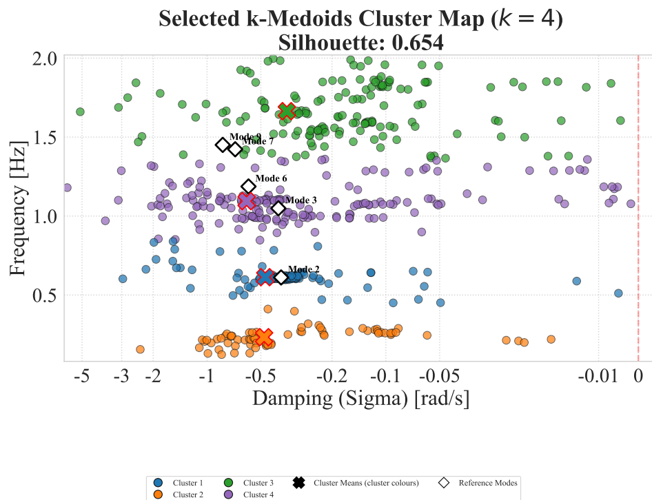
Σχήμα 3.3: Selected cluster map για το πρώτο order sweep και την Περιοχή 3: k -Medoids.
