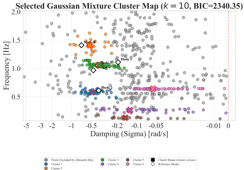
Σχήμα Α'.27: Selected cluster map: GMM (orders2).
