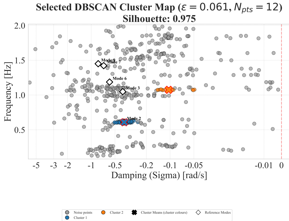
Σχήμα 3.6: Selected cluster map για το πρώτο order sweep και την Περιοχή 3: DBSCAN.
