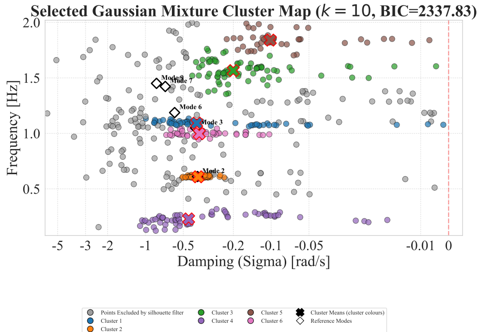
Σχήμα 3.5: Selected cluster map για το πρώτο order sweep και την Περιοχή 3: GMM.
