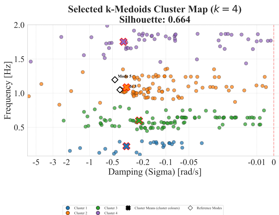
Σχήμα Α'.30: Selected cluster map: k-Medoids (orders2).
