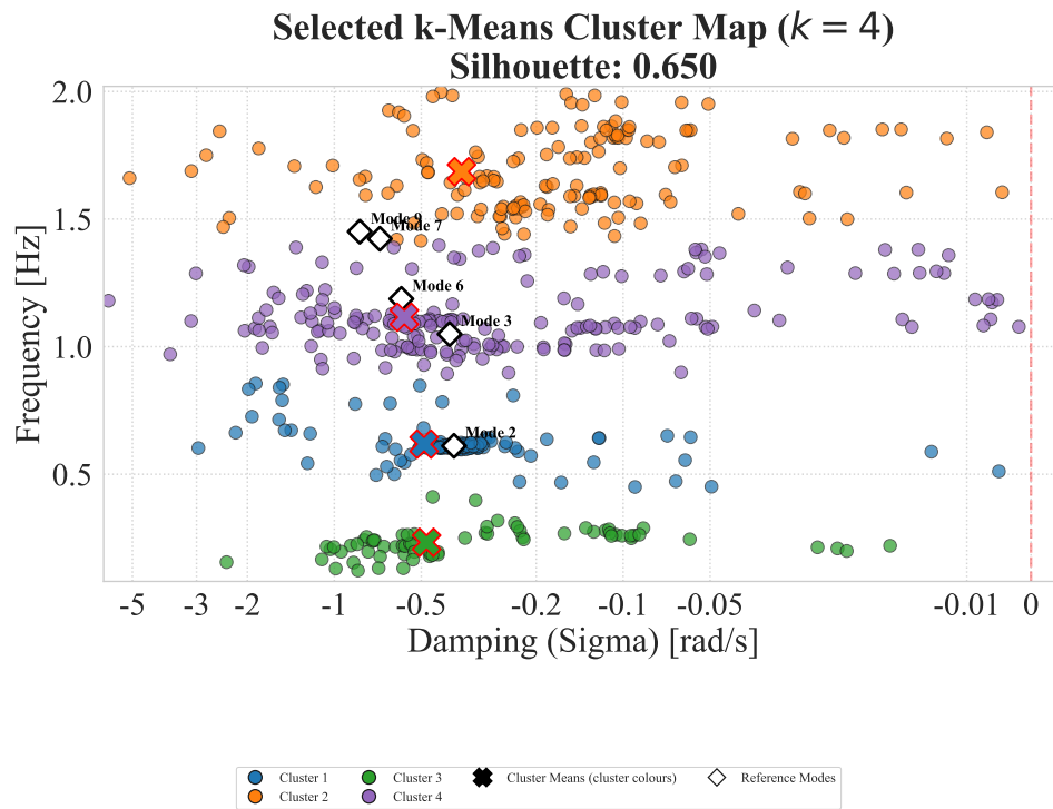
Σχήμα 3.2: Selected cluster map για το πρώτο order sweep και την Περιοχή 3: k -Means.
