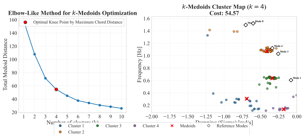
Σχήμα 3.27: Διάγραμμα Elbow του αλγορίθμου k -Medoids για την περιοχή ελέγχου 3 του IEEE 39-Bus System.
