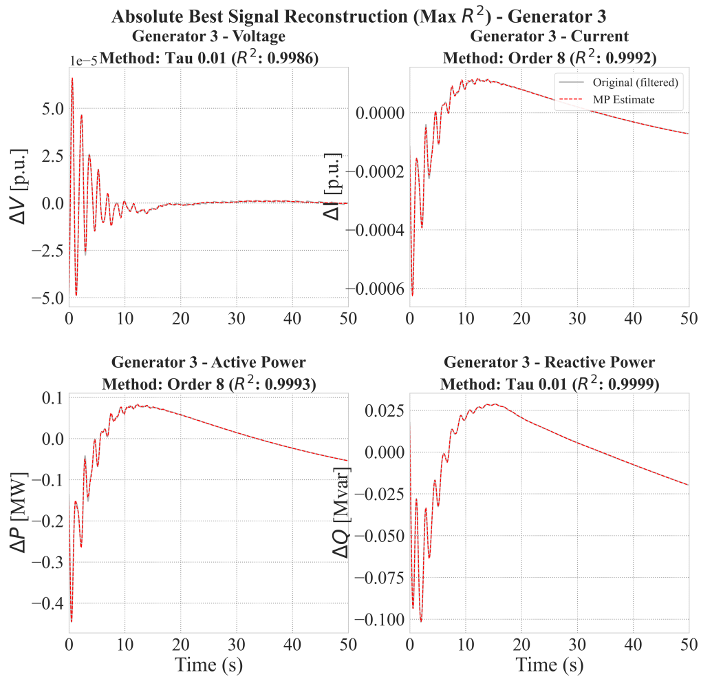
Σχήμα 3.10: Βέλτιστη μαθηματική ανακατασκευή των σημάτων ( V, I, P, Q ) για τη γεννήτρια G_3 του IEEE 39-Bus System με βάση τον μέγιστο συντελεστή προσδιορισμού R^2 .
