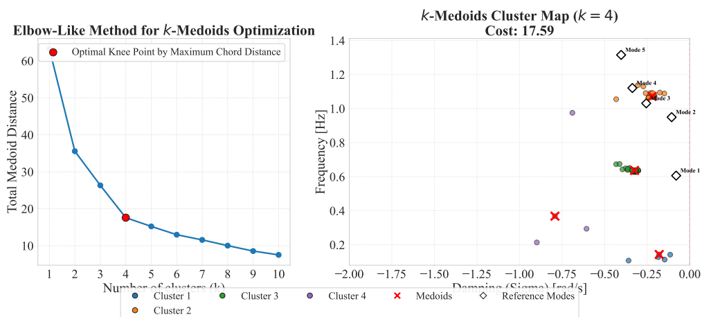
Σχήμα 3.26: Διάγραμμα Elbow του αλγορίθμου k -Medoids για την περιοχή ελέγχου 2 του IEEE 39-Bus System.
