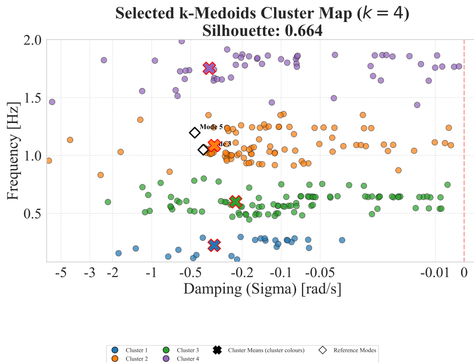
Σχήμα Α'.30: Selected cluster map: k -Medoids (orders2).
