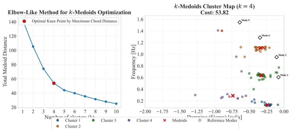
Σχήμα 3.25: Διάγραμμα Elbow του αλγορίθμου k-Medoids για την περιοχή ελέγχου 1 του IEEE 39-Bus System.
