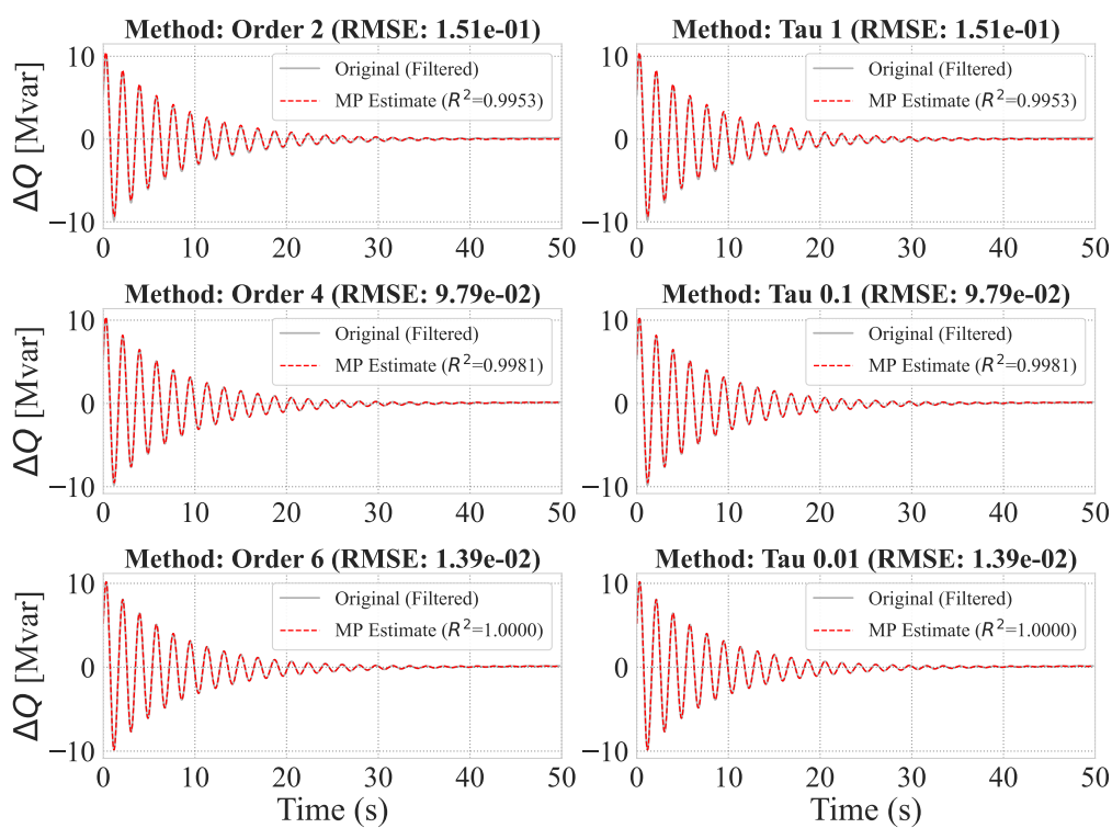
Σχήμα 3.3: Ανακατασκευή σήματος αέργου ισχύος ( Q ) για τη γεννήτρια G_1 του Kundur Two-Area System.
