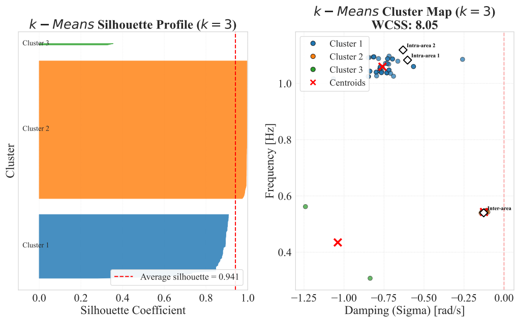
Σχήμα 3.16: Silhouette profile του αλγορίθμου k - Means για k = 3 στο Kundur Two-Area System.
