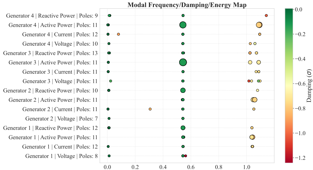
Σχήμα 3.12: Χάρτης Ιδιοτιμών (Bubble Map): Συγκεντρωτική απεικόνιση συχνότητας, απόσβεσης και ενέργειας των ταυτοποιημένων modes.
