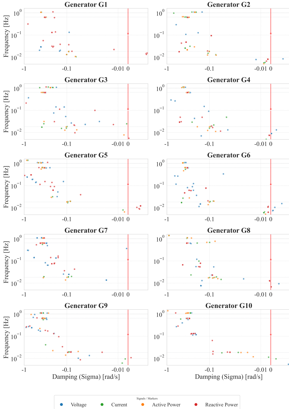
Σχήμα 3.2: Κατανομή ιδιοτιμών (Real Part vs Frequency) για τις γεννήτριες G_1 - G_{10} του IEEE 39-Bus System.
