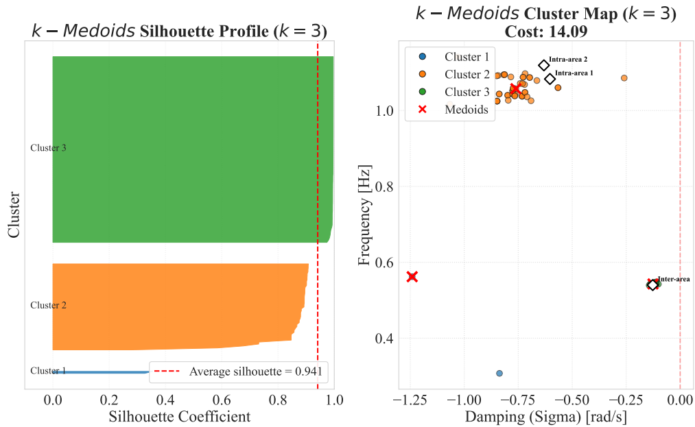
Σχήμα 3.18: Silhouette profile του αλγορίθμου k -Medoids για k = 3 στο Kundur Two-Area System.
