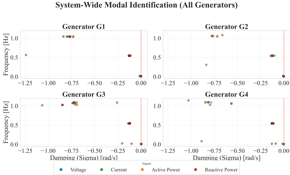
Σχήμα 3.1: Κατανομή ιδιοτιμών (Real Part vs Frequency) για τις γεννήτριες G_1 - G_4 του Kundur Two-Area System.
