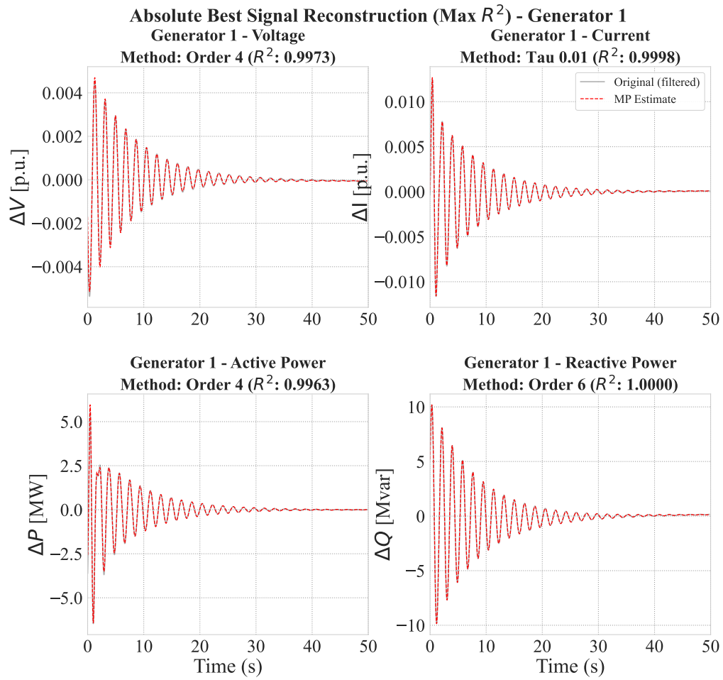
Σχήμα 3.5: Βέλτιστη μαθηματική ανακατασκευή των σημάτων ( V, I, P, Q ) για τη γεννήτρια G_1 του Kundur Two-Area System με βάση τον μέγιστο συντελεστή προσδιορισμού R^2 .
