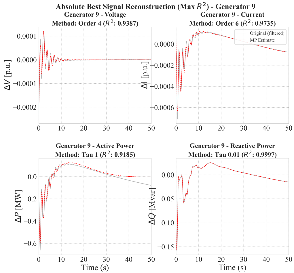
Σχήμα 3.9: Βέλτιστη μαθηματική ανακατασκευή των σημάτων ( V, I, P, Q ) για τη γεννήτρια G_9 του IEEE 39-Bus System με βάση τον μέγιστο συντελεστή προσδιορισμού R^2 .
