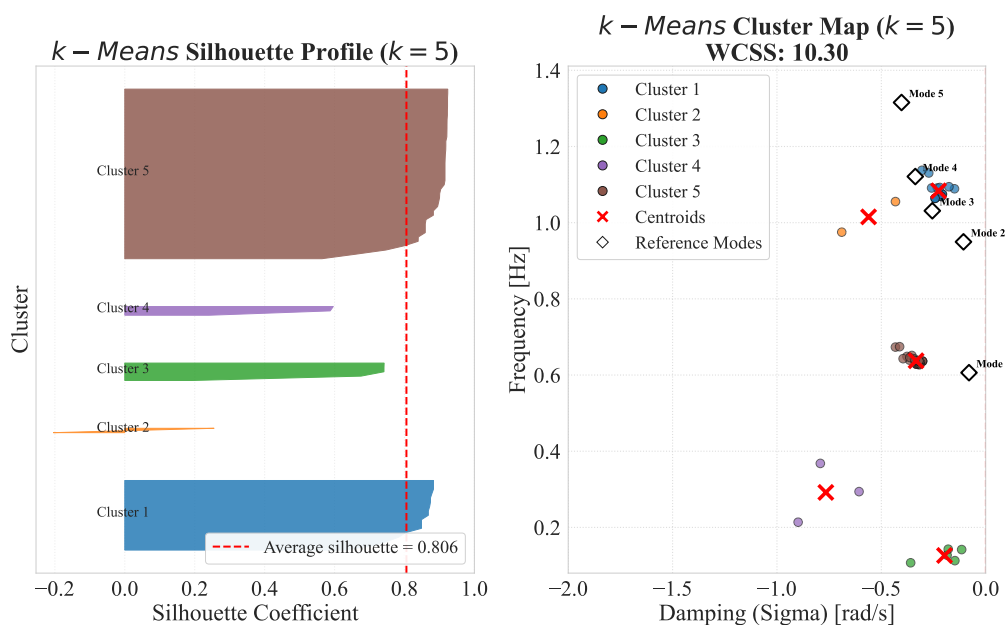
Σχήμα 3.23: Silhouette profile του αλγορίθμου k -Means για k = 5 στην περιοχή ελέγχου 2 του IEEE 39-Bus System.
