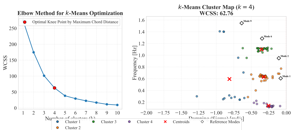
Σχήμα 3.19: Διάγραμμα Elbow του αλγορίθμου k -Means για την περιοχή ελέγχου 1 του IEEE 39-Bus System.
