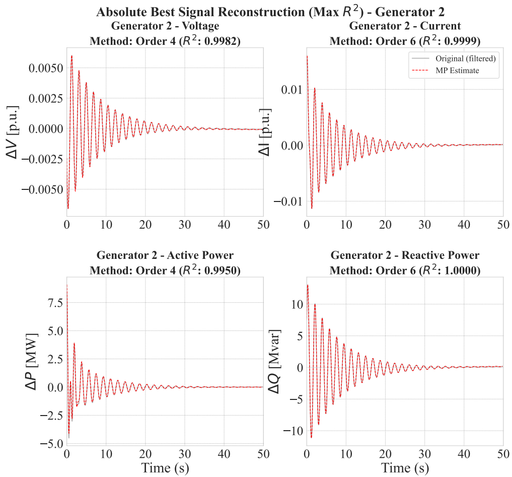
Σχήμα 3.6: Βέλτιστη μαθηματική ανακατασκευή των σημάτων ( V, I, P, Q ) για τη γεννήτρια G_2 του Kundur Two-Area System με βάση τον μέγιστο συντελεστή προσδιορισμού R^2 .
