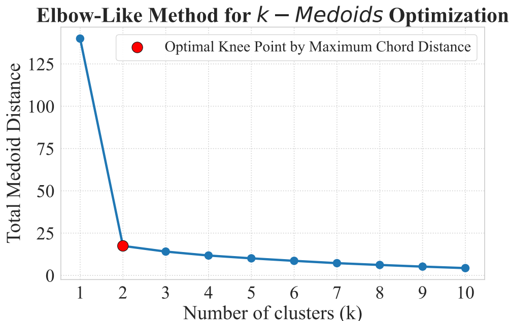
Σχήμα 3.17: Διάγραμμα συνολικού κόστους του αλγορίθμου k-Medoids για το Kundur Two-Area System.
