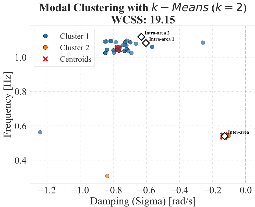
Σχήμα 3.15: Χάρτης ιδιοτιμών του αλγορίθμου k - Means για k = 2 στο Kundur Two-Area System.
