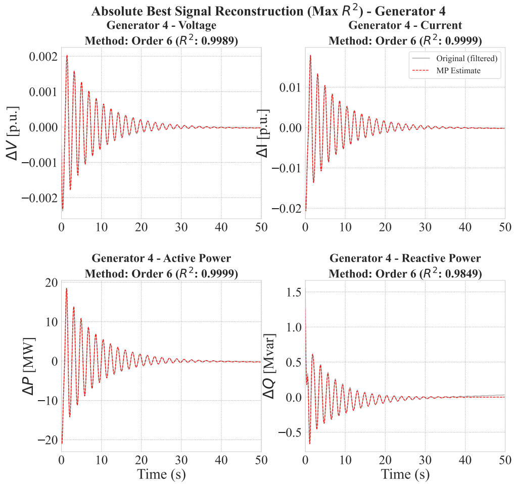
Σχήμα 3.8: Βέλτιστη μαθηματική ανακατασκευή των σημάτων ( V, I, P, Q ) για τη γεννήτρια G_4 του Kundur Two-Area System με βάση τον μέγιστο συντελεστή προσδιορισμού R^2 .
