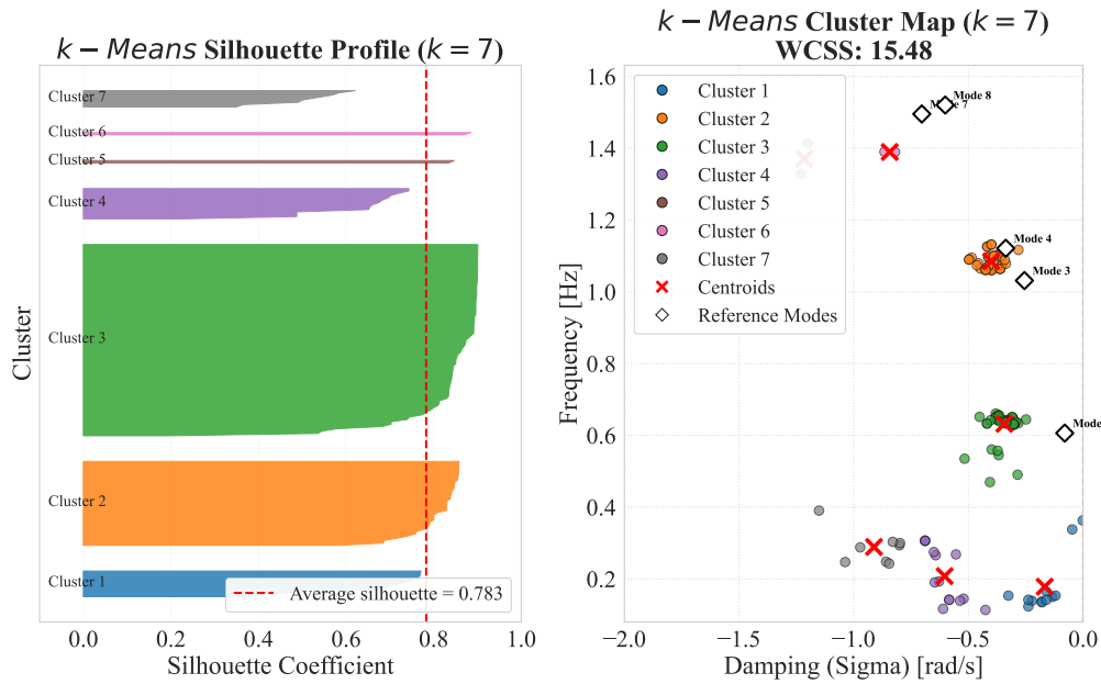
Σχήμα 3.24: Silhouette profile του αλγορίθμου k-Means για k = 7 στην περιοχή ελέγχου 3 του IEEE 39-Bus System.
