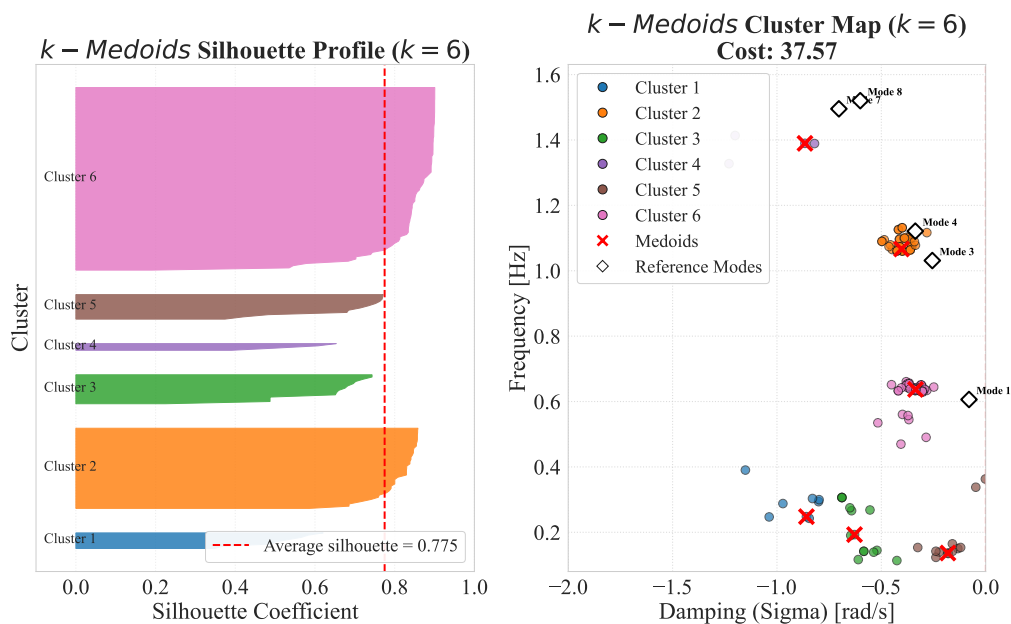
Σχήμα 3.30: Silhouette profile του αλγορίθμου k -Medoids για k = 6 στην περιοχή ελέγχου 3 του IEEE 39-Bus System.
