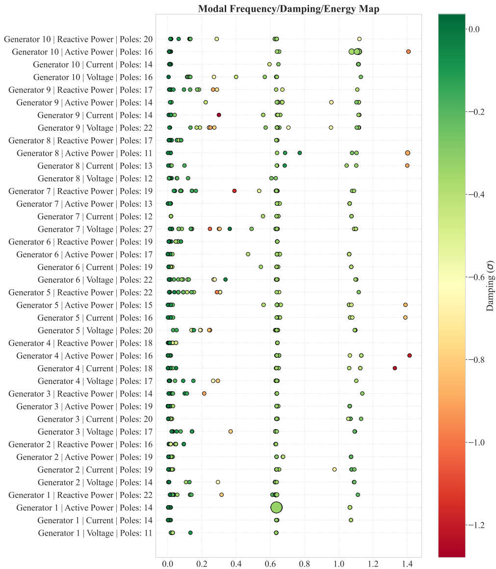
Σχήμα 3.13: Χάρτης Ιδιοτιμών (Bubble Map): Συγκεντρωτική απεικόνιση συχνότητας, απόσβεσης και ενέργειας των ταυτοποιημένων modes.
