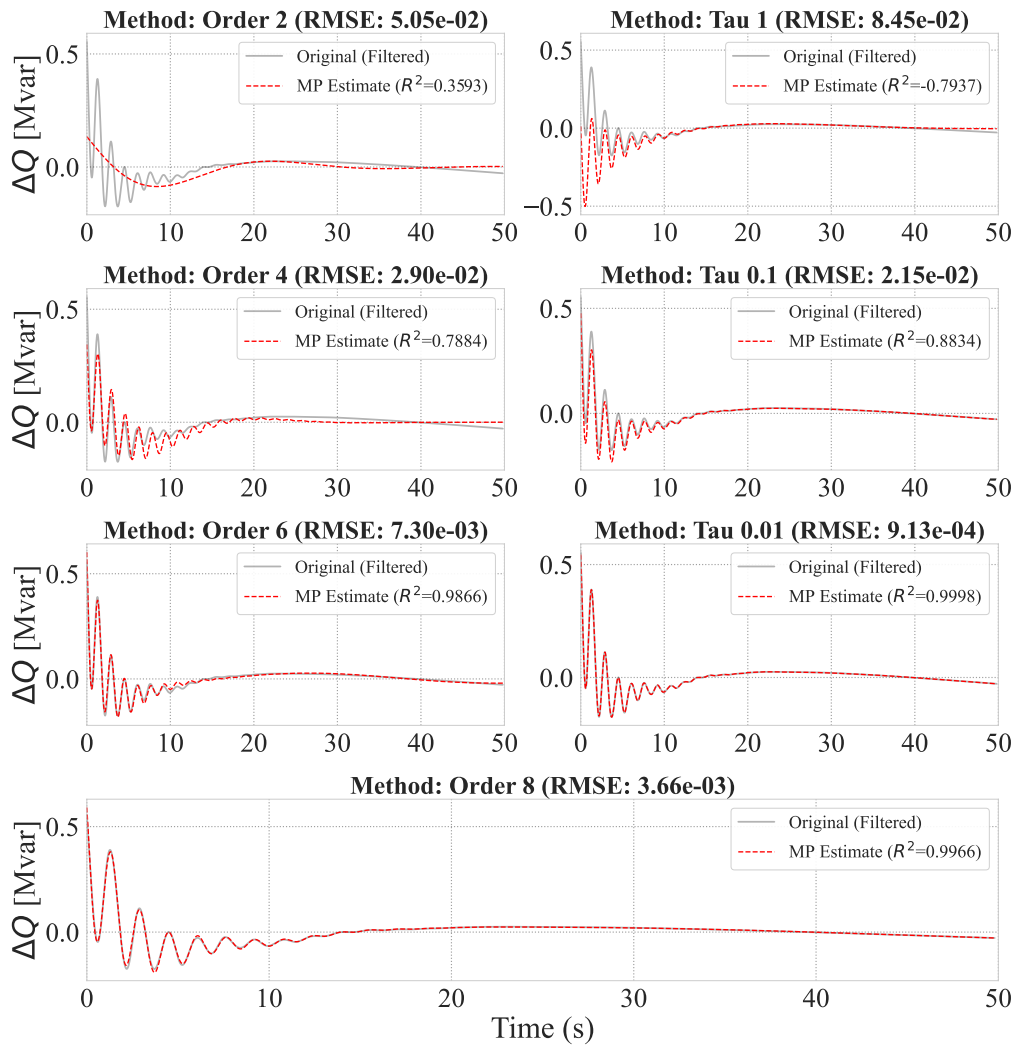
Σχήμα 3.4: Ανακατασκευή σήματος αέργου ισχύος ( Q ) για τη γεννήτρια G_1 του IEEE 39-Bus System.
