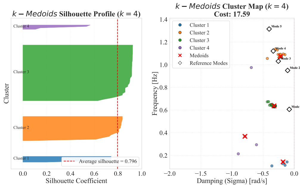
Σχήμα 3.29: Silhouette profile του αλγορίθμου k -Medoids για k = 4 στην περιοχή ελέγχου 2 του IEEE 39-Bus System.
