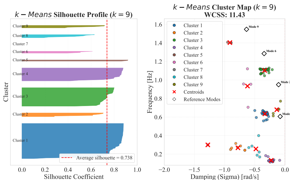
Σχήμα 3.22: Silhouette profile του αλγορίθμου k -Means για k = 9 στην περιοχή ελέγχου 1 του IEEE 39-Bus System.
