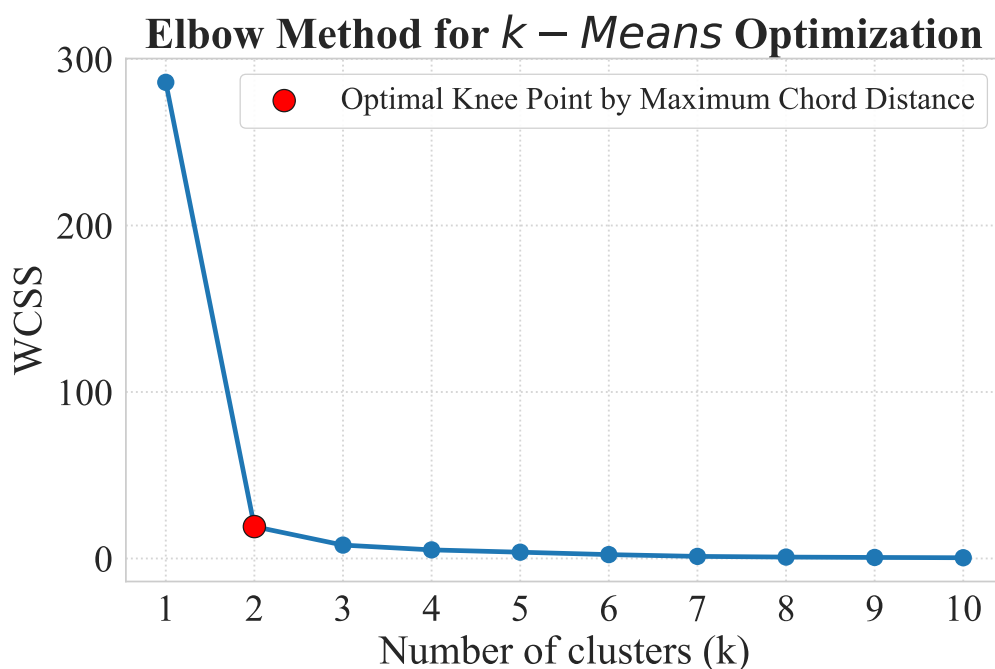
Σχήμα 3.14: Διάγραμμα Elbow του αλγορίθμου k-Means για το Kundur Two-Area System .
