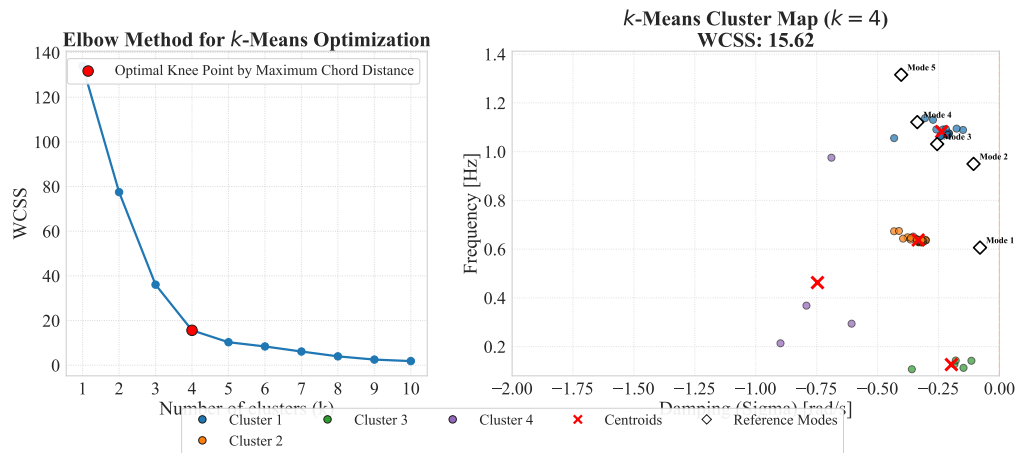
Σχήμα 3.20: Διάγραμμα Elbow του αλγορίθμου k -Means για την περιοχή ελέγχου 2 του IEEE 39-Bus System.
