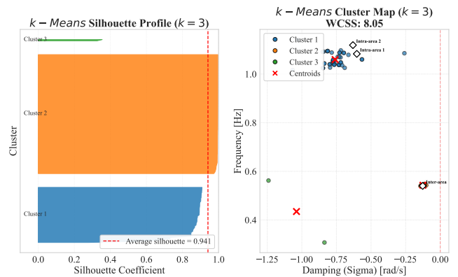
Fig. 16. Silhouette profile του αλγορίθμου k-Means για k = 3 στο Kundur Two-Area System.
