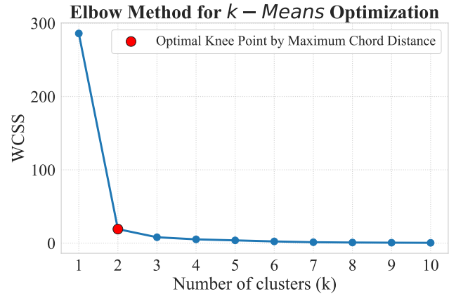
Fig. 14. Διάγραμμα Elbow του αλγορίθμου k-Means για το Kundur Two-Area System.
