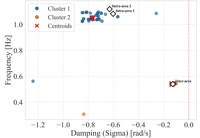
Fig. 15. Χάρτης ιδιοτιμών του αλγορίθμου k-Means για k = 2 στο Kundur Two-Area System.
