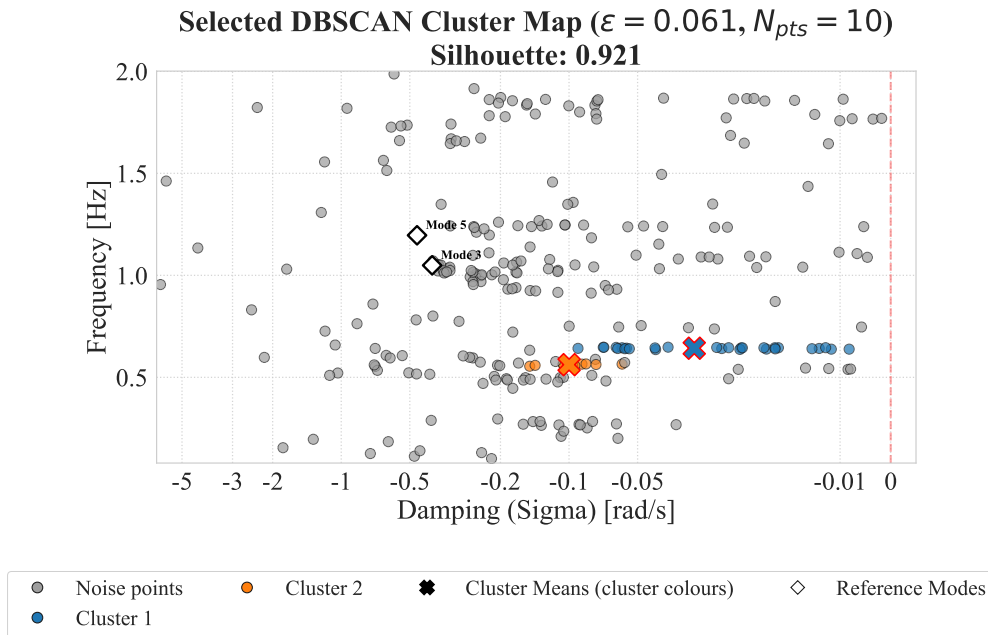
Σχήμα Α'.31: Selected cluster map: DBSCAN (orders2).
