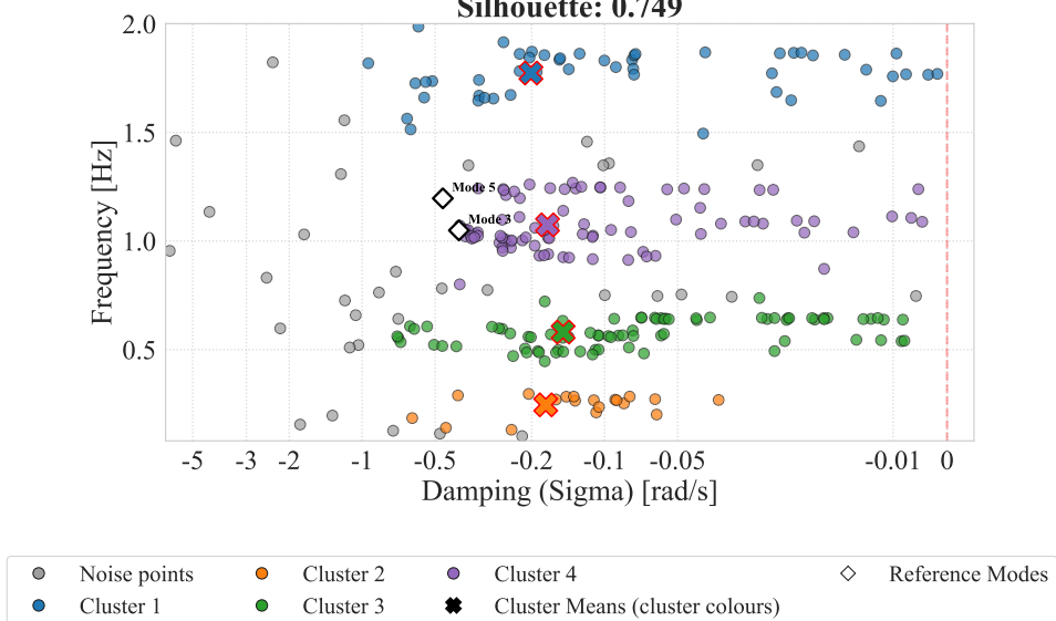
Σχήμα Α'.33: Selected cluster map: HDBSCAN (orders2).
