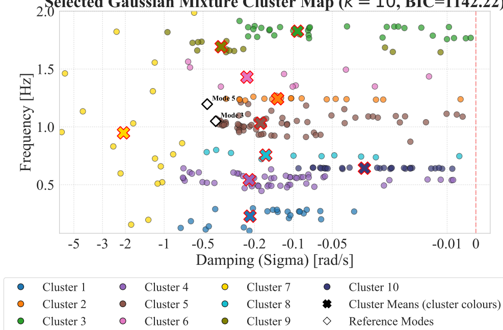
Σχήμα Α'.34: Selected cluster map: GMM (orders2).
