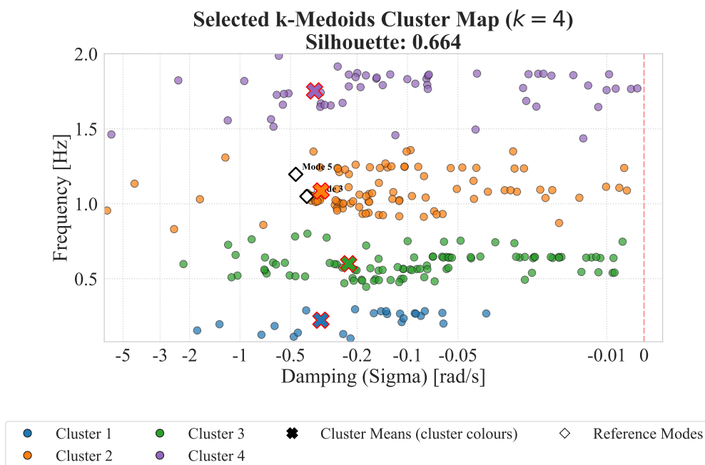
Σχήμα Α'.30: Selected cluster map: k-Medoids (orders2).
