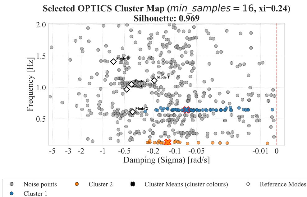
Σχήμα Α'.25: Selected cluster map: OPTICS (orders2).
