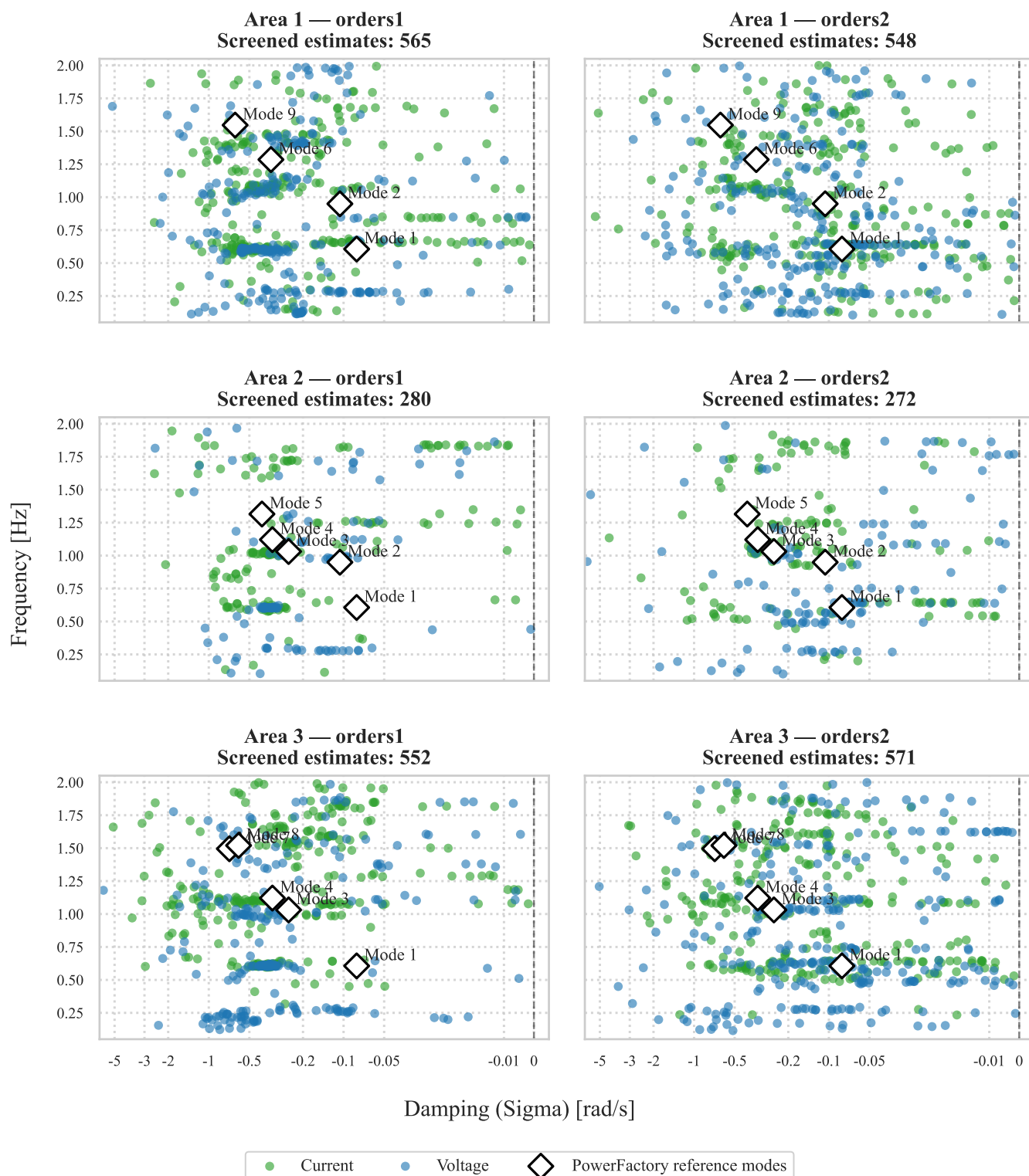
Σχήμα 3.1: Screened εκτιμήσεις N4SID στο επίπεδο (\sigma, f) ανά order sweep και περιοχή ελέγχου. Οι χρωματισμοί διακρίνουν τα σήματα τάσης και ρεύματος, ενώ οι λευκοί ρόμβοι δηλώνουν τους ρυθμούς αναφοράς του PowerFactory του Πίνακα 2.1.
