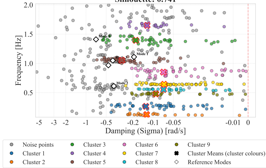
Σχήμα Α'.26: Selected cluster map: HDBSCAN (orders2).
