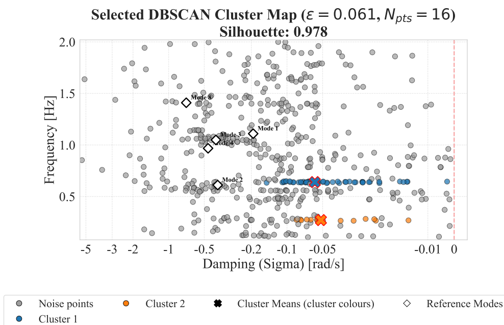
Σχήμα Α'.24: Selected cluster map: DBSCAN (orders2).
