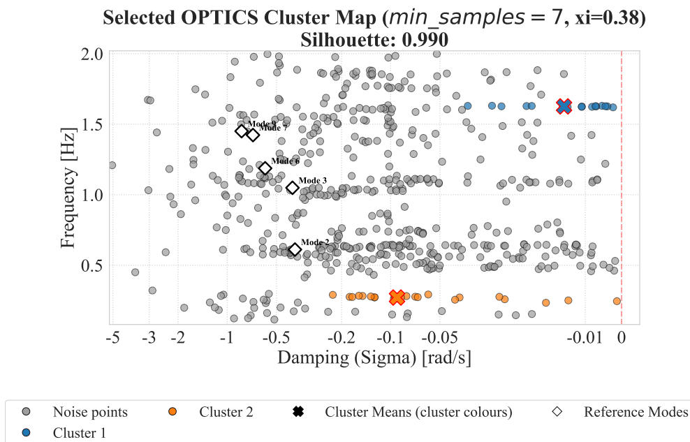
Σχήμα Α'.39: Selected cluster map: OPTICS (orders2).
