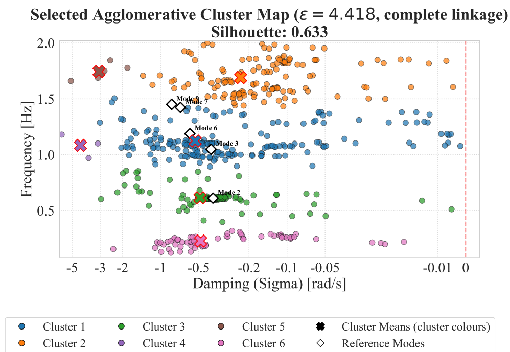
Σχήμα 3.8: Selected cluster map για το πρώτο order sweep και την Περιοχή 3: Agglomerative Hierarchical Clustering.
