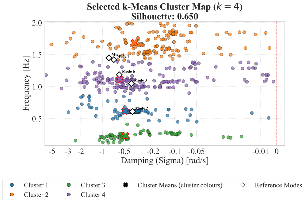
Σχήμα 3.2: Selected cluster map για το πρώτο order sweep και την Περιοχή 3: k-Means.
