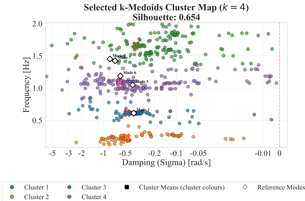
Σχήμα 3.3: Selected cluster map για το πρώτο order sweep και την Περιοχή 3: k-Medoids.
