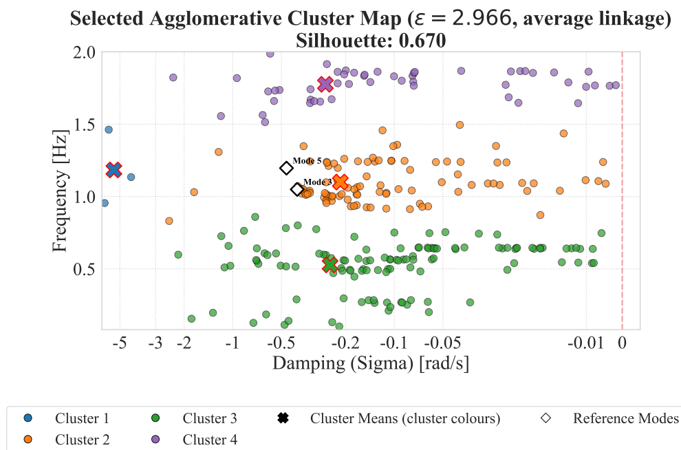
Σχήμα Α'.35: Selected cluster map: Agglomerative Hierarchical Clustering (orders2).
