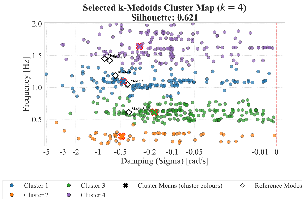
Σχήμα Α'.37: Selected cluster map: k-Medoids (orders2).
