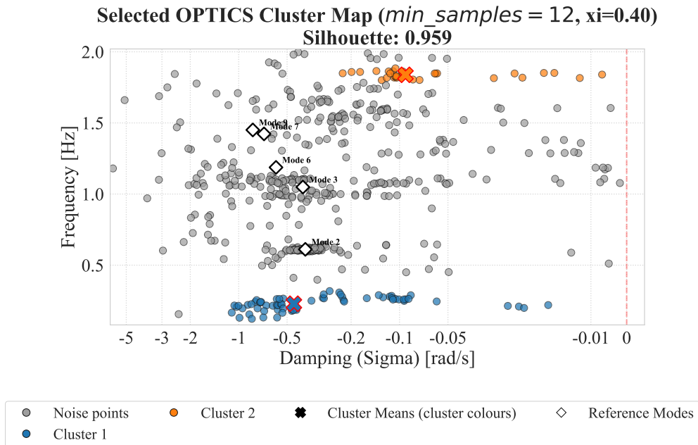
Σχήμα 3.7: Selected cluster map για το πρώτο order sweep και την Περιοχή 3: OPTICS.
