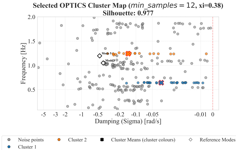
Σχήμα Α'.32: Selected cluster map: OPTICS (orders2).
