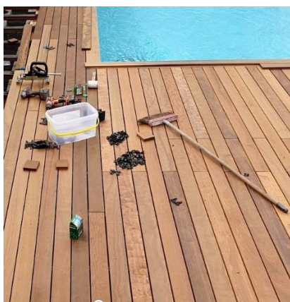
Ci-dessus lame de terrasse en itauba 21 x 100 mm clipsée sans vis apparentes
