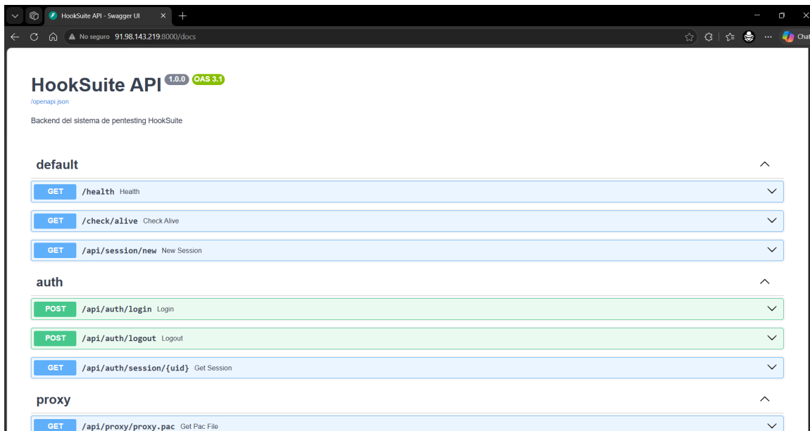
Figura 7: RNF-07 / PR-16 — la documentación Swagger (/docs) queda abierta a cualquiera, exponiendo las 40 operaciones de la API, incluidas las que lanzan tráfico contra terceros.
