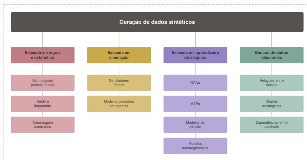
Figura 1: Técnicas de geração de dados sintéticos. Fonte: Elaboração própria
