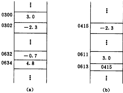
图 1.6 复数存储结构示意图 (a) 顺序存储结构; (b) 链式存储结构
