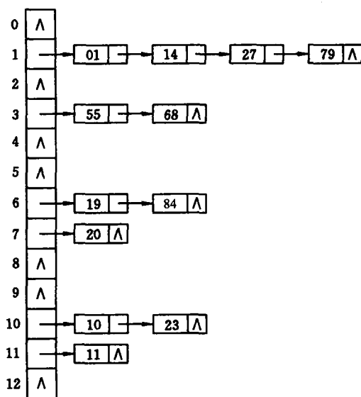
图 9.26 链地址法处理冲突时的哈希表
