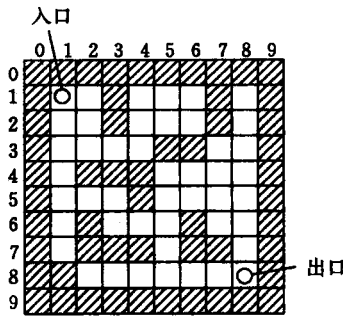
图 3.4 迷宫
