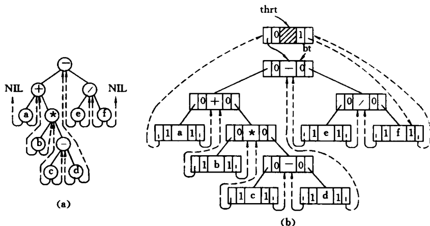
图 6.11 线索二叉树及其存储结构
