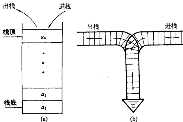
图 3.1 栈
