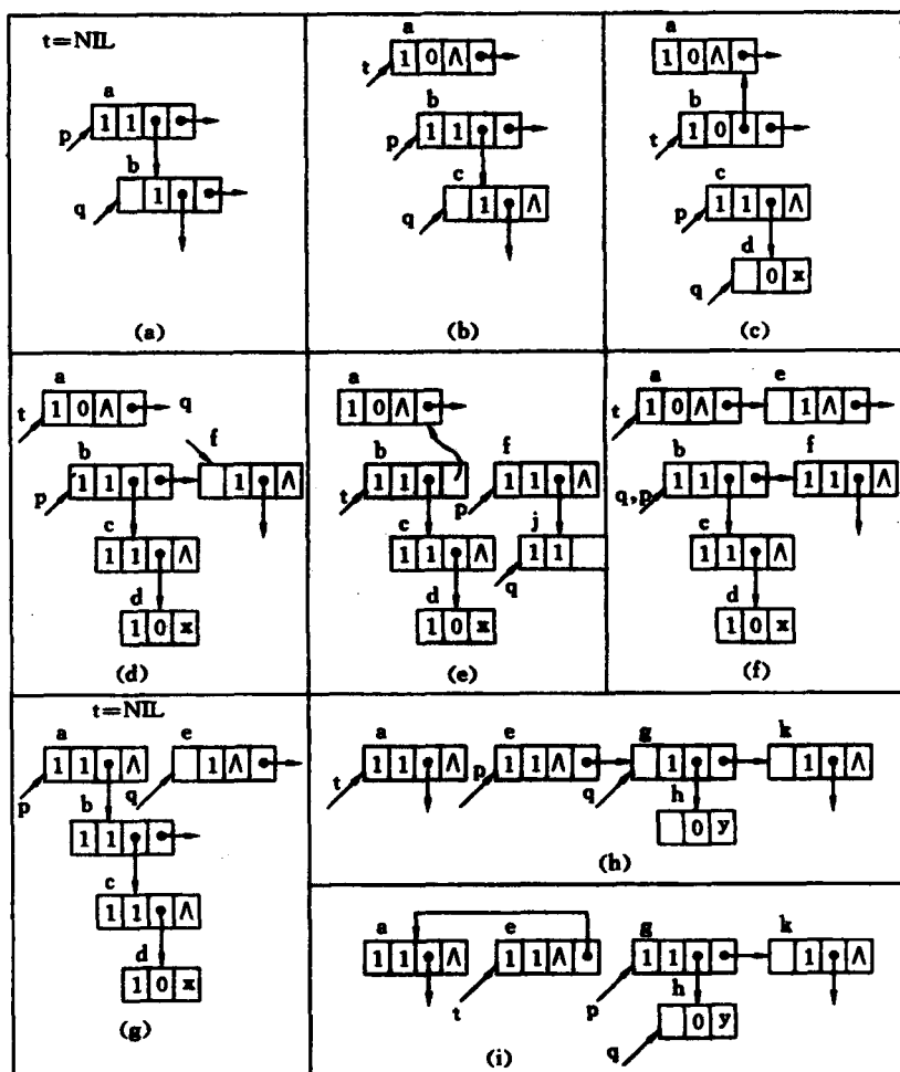
图 8.11 遍历广义表
